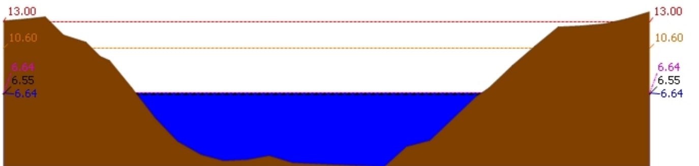
▲ ระดับปัจจุบัน --- ระดับวิกฤติ --- ระดับฝายระวัง ---- เมื่อกวาน 7:00 น. - - - - คาคตการลลลวงหน้า 1 วัน สถานี 120106T แม่น้ำป่าสักที่ อ.เสาไห้ ต.ศาลารี่ไทย อ.เสาไห้ จ.สระบุรี ระดับน้ำ 6.64 ม.รทก.
