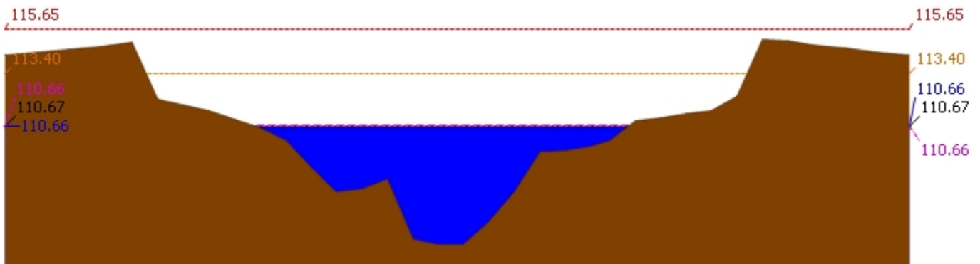
▲ ระดับปัจจุบัน --- ระดับวิกฤติ --- ระดับฝายระวัง ---- เมื่อกวาน 7:00 น. - - - - คาคตการลลลวงหน้า 1 วัน สถานี 120107T แม่น้ำป่าสักที่ อ.เมืองเพชรบูรณ์ ต.นาป่า อ.เมือง จ.เพชรบูรณ์ ระดับน้ำ 110.66 ม.รทก.
