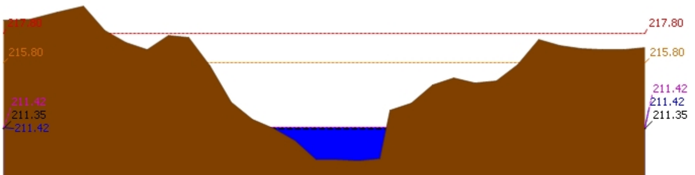
▲ ระดับปัจจุบัน --- ระดับวิกฤติ --- ระดับฝายระวัง ---- เมื่อกวาน 7:00 น. - - - - คาคตการลลลวงหน้า 1 วัน สถานี 120205T แม่น้ำป่าสักที่บ้านลุ่มกะทาด ต.ศิลา อ.หล่มเก่า จ.เพชรบูรณ์ ระดับน้ำ 211.42 ม.รทก.
