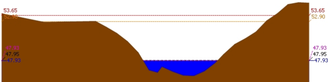
▲ ระดับปัจจุบัน --- ระดับวิกฤติ --- ระดับเฝ้าระวัง ---- เมื่อกาน 7:00 น. - - - - คาดการณ์ล่วงหน้า 1 วัน สถานี 120113T แม่น้ำป่าสักที่บ้านเขาค้าง ต.คลองกระจิง อ.ศรีเทพ จ.เพชรบูรณ์ ระดับน้ำ 47.93 ม.รทก.
