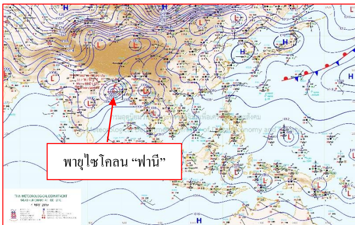
แผนที่อากาศ วันที่ ๔ พ.ค. ๒๕๖๒ เวลา ๐๗.๐๐ น.
