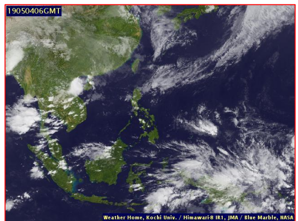
ภาพถ่ายดาวเทียม วันที่ ๔ พ.ค. ๒๕๖๒ เวลา ๑๓.๐๐ น.
