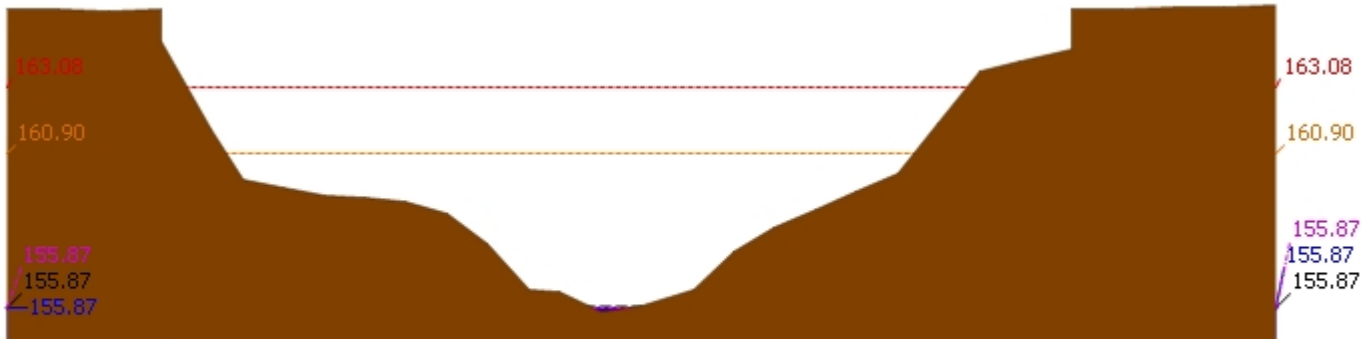
▲ ระดับปัจจุบัน --- ระดับวิกฤติ --- ระดับเฟิาระวัง ---- เมื่อวาน 7:00 น. - - - - คาคตการล้ลวงหน้า 1 วัน สถานี 120105T แม่น้ำป่าสักที่บ้านวังมเสหนือ ต.ทำอึบุญ อ.หล่มสัก จ.เพชรบูรณ์ ระดับน้ำ 155.87 ม.รทก.
