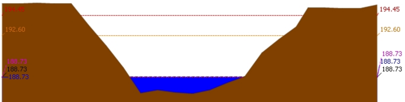
▲ ระดับปัจจุบัน --- ระดับวิกฤติ --- ระดับเฝ้าระวัง ---- เมื่อวาน 7:00 น. - - - - - คาดการณ์ล่วงหน้า 1 วัน สถานี 120901T ห้วยมวกเหล็กที่ อ.มวกเหล็ก ต.มวกเหล็ก อ.มวกเหล็ก จ.สระบุรี ระดับน้ำ 188.73 ม.รทก.
