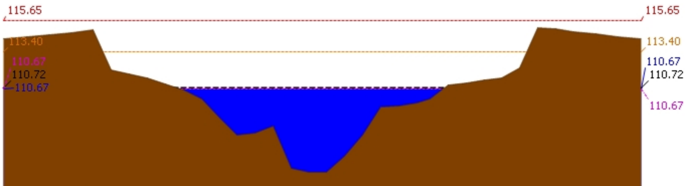
▲ ระดับปัจจุบัน --- ระดับวิกฤติ --- ระดับเฟิาระวัง ---- เมื่อกาน 7:00 น. - - - - คาคการล่ลวงหน้า 1 วัน สถานี 120107T แม่น้ำป่าสักที่ อ.เมืองเพชรบูรณ์ ต.นาป่า อ.เมือง จ.เพชรบูรณ์ ระดับน้ำ 110.67 ม.รทก.
