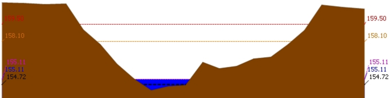
▲ ระดับปัจจุบัน --- ระดับวิกฤติ --- ระดับเฟิาระวัง ---- เมื่อวาน 7:00 น. - - - - คาคตการล้ลวงหน้า 1 วัน สถานี 120305T หัวน้ำพุทที่ อ.หล่มเก่า ต.หล่มเก่า อ.หล่มเก่า จ.เพชรบูรณ์ ระดับน้ำ 155.11 ม.รทก.
