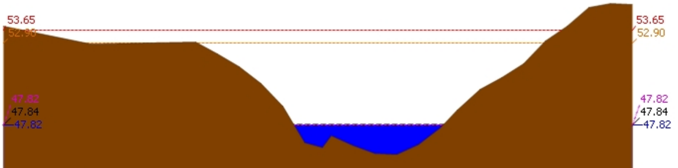
▲ ระดับปัจจุบัน --- ระดับวิกฤติ --- ระดับเฝ้าระวัง ---- เมื่อวาน 7:00 น. - - - - - คาดการณ์ล่วงหน้า 1 วัน สถานี 120113T แม่น้ำป่าสักที่บ้านเขาค้าง ต.คลองกระจิง อ.ศรีเทพ จ.เพชรบูรณ์ ระดับน้ำ 47.82 ม.รทก.
