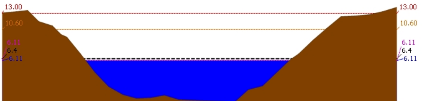
▲ ระดับปัจจุบัน --- ระดับวิกฤติ --- ระดับเฟิาระวัง ---- เมื่อกาน 7:00 น. - - - - คาคการล่ลวงหน้า 1 วัน สถานี 120106T แม่น้ำป่าสักที่ อ.เสาไห้ ต.ศาลาริไทย อ.เสาไห้ จ.สระบุรี ระดับน้ำ 6.11 ม.รทก.
