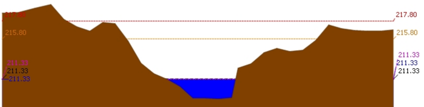
▲ ระดับปัจจุบัน --- ระดับวิกฤติ --- ระดับเฟิาระวัง ---- เมื่อกาน 7:00 น. - - - - คาคการล่ลวงหน้า 1 วัน สถานี 120205T แม่น้ำป่าสักที่ บ้านอู่กะทาด ต.ศิลา อ.หล่มเก่า จ.เพชรบูรณ์ ระดับน้ำ 211.33 ม.รทก.
