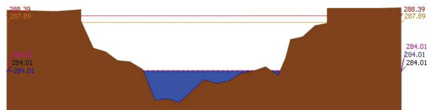
รายงานสถานการณ์น้ำลุ่มน้ำวัง วันที่ 5 มิถุนายน 2562
