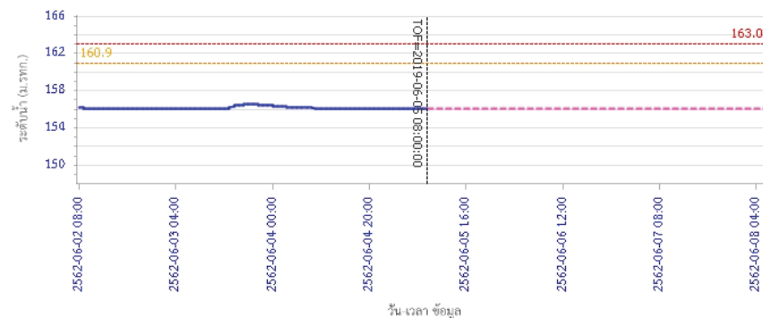
รายงานสถานการณ์น้ำลุ่มน้ำป่าสัก วันที่ 5 มิถุนายน 2562
