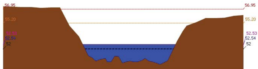
รายงานสถานการณ์น้ำลุ่มน้ำสะแกกรัง วันที่ 5 มิถุนายน 2562
