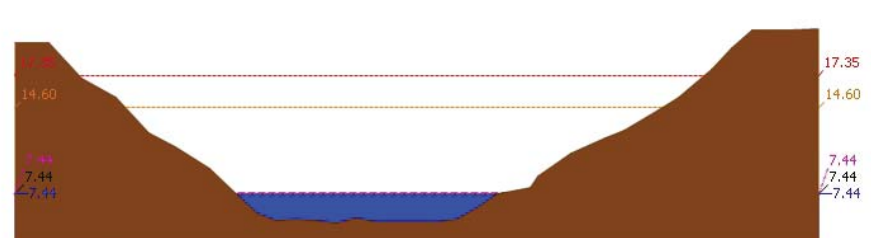
รายงานสถานการณ์น้ำลุ่มน้ำป่าสัก วันที่ 5 มิถุนายน 2562
