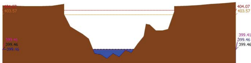
รายงานสถานการณ์น้ำลุ่มน้ำวัง วันที่ 5 มิถุนายน 2562
