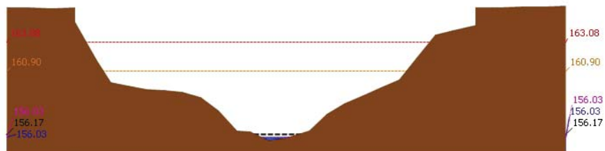
รายงานสถานการณ์น้ำลุ่มน้ำป่าสัก วันที่ 5 มิถุนายน 2562
