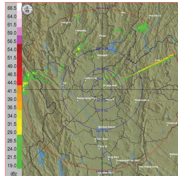
ภาพเรดาร์ตรวจอากาศ “พิษณุโลก” ณ วันที่ 5 มิถุนายน 2562 (ที่มา : กรมอุตุนิยมวิทยา)
