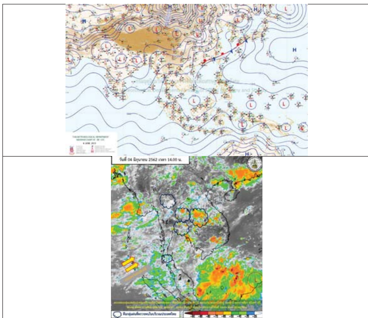
รูปที่ 1 พยากรณ์อากาศ วันที่ 5 มิ.ย. 2562
