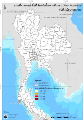
วันที่ 5 มิ.ย. 2562 (19:00 น.)
