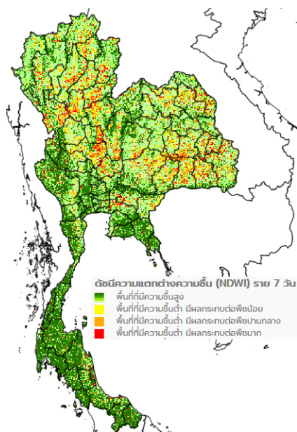
แผนที่ดาวเทียมของ Gistda (30 พ.ค. – 5 มิ.ย. 62)
