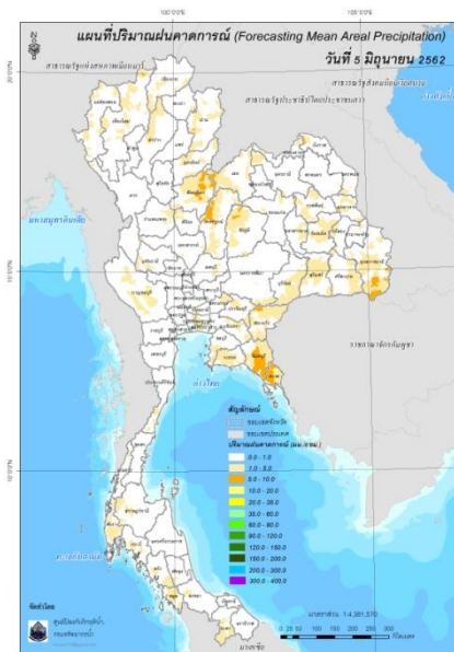
ปริมาณฝนคาดการณ์ในวันที่ 5 มิถุนายน 2562
