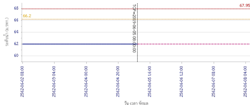
รายงานสถานการณ์น้ำลุ่มน้ำสะแกกรัง วันที่ 5 มิถุนายน 2562
