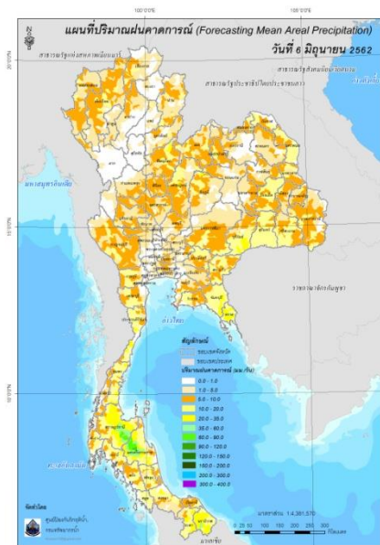
ปริมาณฝนคาดการณ์ในวันที่ 6 มิถุนายน 2562
