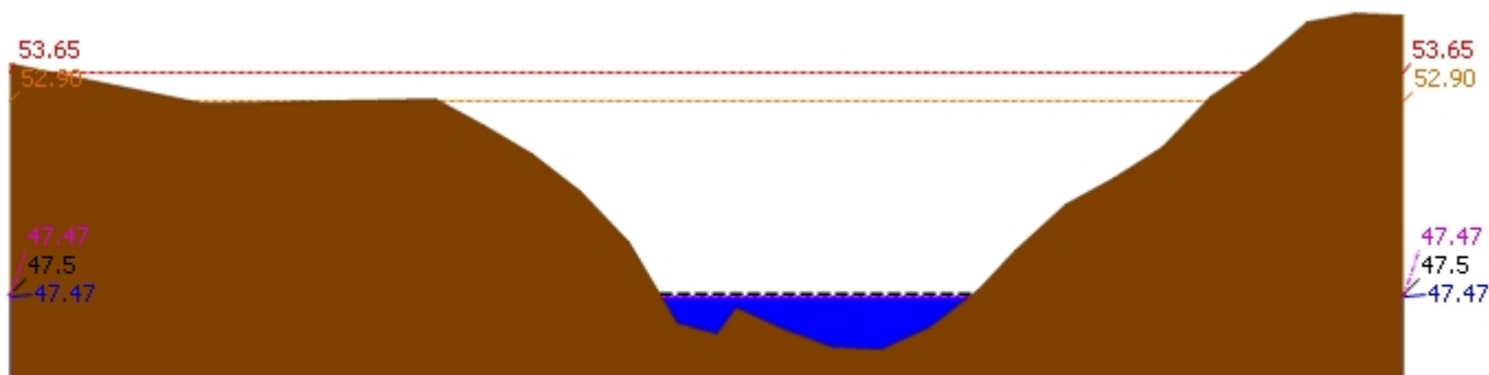
▲ ระดับปัจจุบัน --- ระดับวิกฤติ --- ระดับฝายระวัง ---- เมื่อวาน 7:00 น. - - - - คาดการณ์ล่วงหน้า 1 วัน สถานี 120113T แม่น้ำป่าสักที่บ้านเขาค้าง ต.คลองกระจิง อ.ศรีเทพ จ.เพชรบูรณ์ ระดับน้ำ 47.47 ม.รทก.
