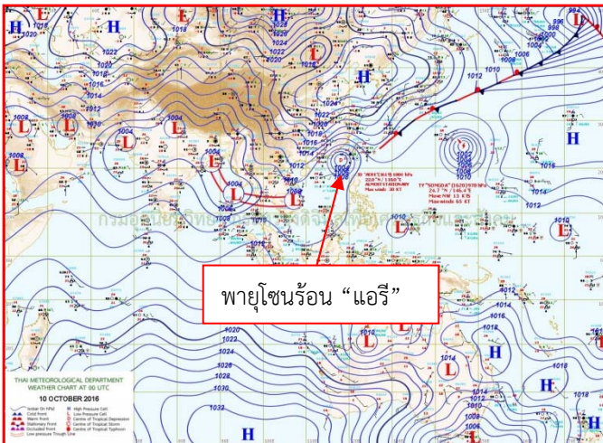
แผนที่อากาศ วันที่ ๑๐ ต.ค. ๒๕๕๙ เวลา ๐๗.๐๐ น.
