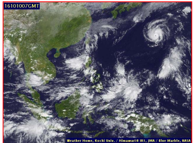
ภาพถ่ายจากดาวเทียม วันที่ ๑๐ ต.ค. ๒๕๕๙ เวลา ๑๓.๐๐ น.
