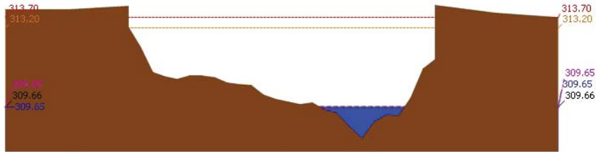
รายงานสถานการณ์น้ำลุ่มน้ำปิง วันที่ 18 มิถุนายน 2562
