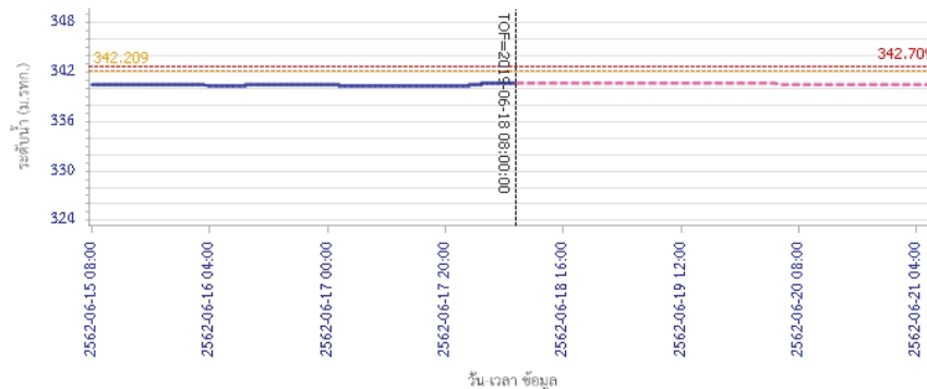
รายงานสถานการณ์น้ำลุ่มน้ำวัง วันที่ 18 มิถุนายน 2562
