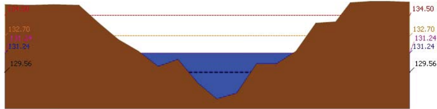
▲ ระดับปัจจุบัน --- ระดับวิกฤติ --- ระดับเฝ้าระวัง --- เมื่อก่อน 7:00 น. --- คาดการณ์ล่วงหน้า 1 วัน สถานี 120111T แม่น้ำป่าสักที่บ้านจางวาง ต.ลานบ่า อ.หล่มสัก จ.เพชรบูรณ์ ระดับน้ำ 131.24 ม.รทก.
