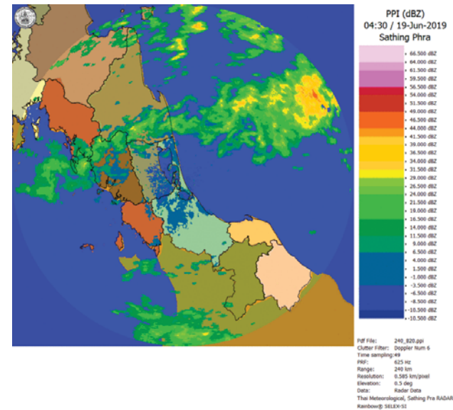
ภาพเรดาร์ตรวจอากาศ “สทิทพะระ” ณ วันที่ 19 มิถุนายน 2562 (ที่มา : กรมอุตุนิยมวิทยา)
