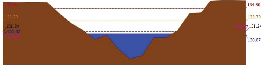
▲ ระดับปัจจุบัน --- ระดับวิกฤติ --- ระดับเฝ้าระวัง --- เมื่อก่อน 7:00 น. --- คาดการณ์ล่วงหน้า 1 วัน สถานี 120111T แม่น้ำป่าสักที่บ้านจางวาง ต.ลานบ่า อ.หล่มสัก จ.เพชรบูรณ์ ระดับน้ำ 130.87 ม.รทก.
