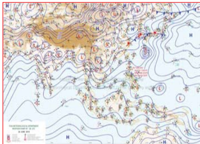
แผนที่อากาศ วันที่ 27 มิ.ย. 2562 เวลา 07.00 น.
