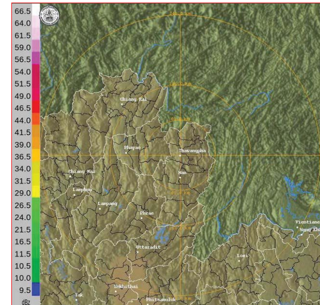
ภาพเรดาร์ตรวจอากาศ “น่าน” ณ วันที่ 27 มิถุนายน 2562 (ที่มา : กรมอุตุนิยมวิทยา)
