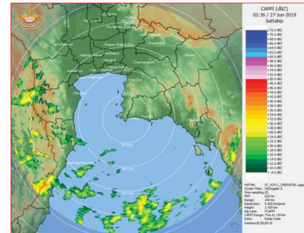
ภาพเรดาร์ตรวจอากาศ “สถานีสดหีบ” ณ วันที่ 27 มิถุนายน 2562 เวลา 09.36 น. (ที่มา : กรมอุตุนิยมวิทยา)
