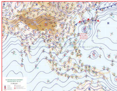
แผนที่อากาศ วันที่ 27 มิ.ย. 2562 เวลา 07.00 น.
