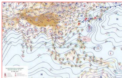
แผนที่อากาศ วันที่ 27 มิ.ย. 2562 เวลา 07.00 น.
