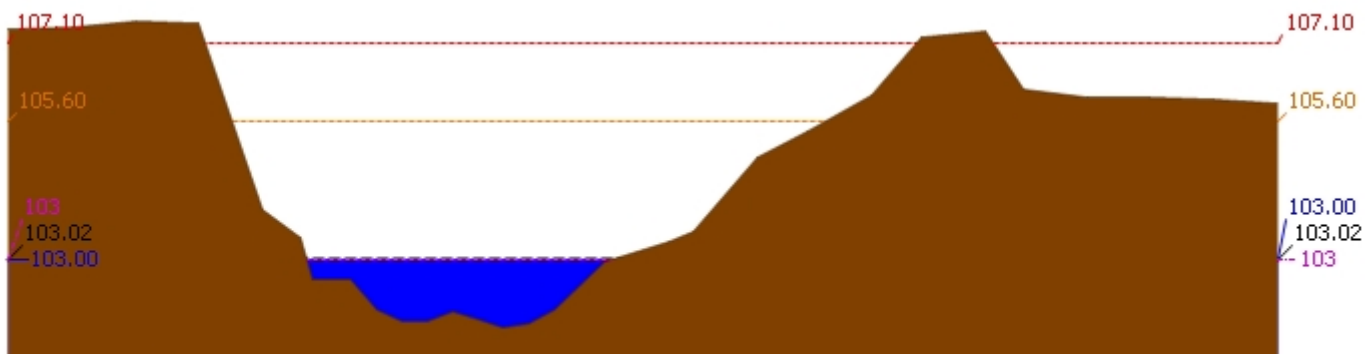
▲ ระดับปัจจุบัน --- ระดับวิกฤติ --- ระดับเฝ้าระวัง ---- เมื่อนาน 7:00 น. - - - - - คาดการณ์ล่วงหน้า 1 วัน สถานี 110402T ฝายทับเสลาที่บ้านนาไร่เดียว ต.ลานสัก อ.ลานสัก จ.อุทัยธานี ระดับน้ำ 103.00 ม.รทก.
