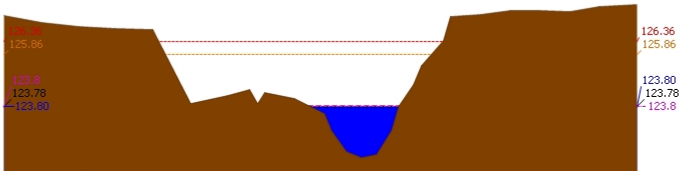
▲ ระดับปัจจุบัน --- ระดับวิกฤติ --- ระดับเฝ้าระวัง ---- เมื่อนาน 7:00 น. - - - - - คาดการณ์ล่วงหน้า 1 วัน สถานี 110401T ฝายทับเสลาที่บ้านบึงอ้ายเจียม ต.ระบำ อ.ลานสัก จ.อุทัยธานี ระดับน้ำ 123.80 ม.รทก.
