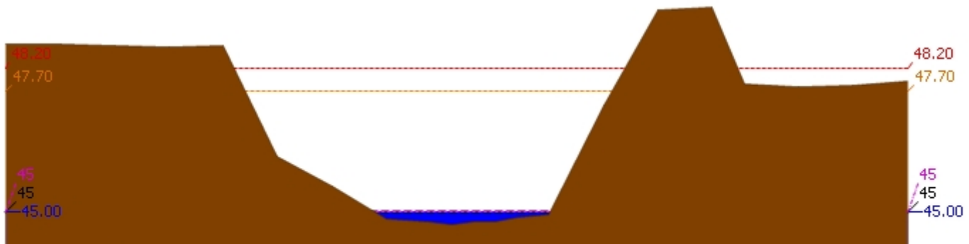
▲ ระดับปัจจุบัน --- ระดับวิกฤติ --- ระดับเฝ้าระวัง ---- เมื่อนาน 7:00 น. - - - - - คาดการณ์ล่วงหน้า 1 วัน สถานี 110303T คลองโพธิ์ที่บ้านทุ่งสงบ ต.ไม้เขี้ยว อ.สว่างอารมณ์ จ.อุทัยธานี ระดับน้ำ 45.00 ม.รทก.
