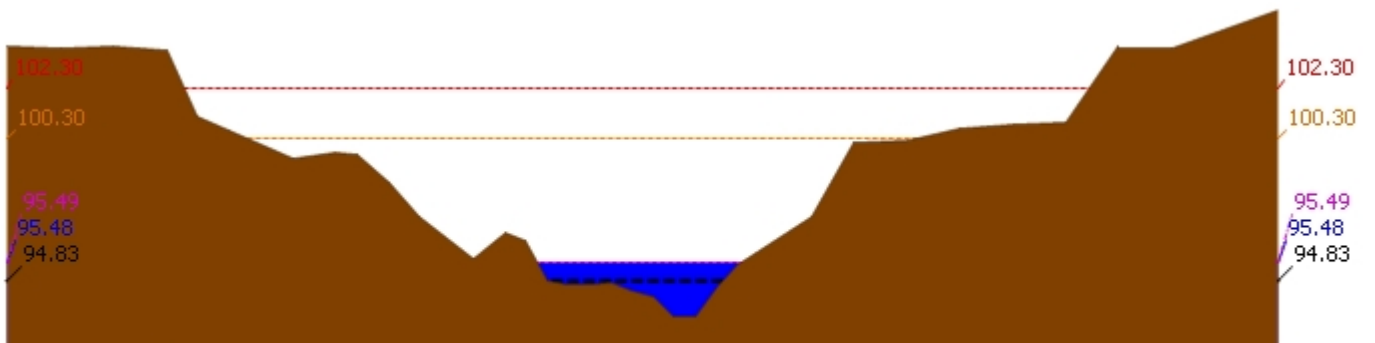
▲ ระดับปัจจุบัน --- ระดับวิกฤติ --- ระดับฝายระวัง ---- เมื่อวาน 7:00 น. - - - - คาดการณ์ล่วงหน้า 1 วัน สถานี 120112T แม่น้ำป่าสักที่บ้านหนองแหวน อ.วังมะข่อ จ.เพชรบูรณ์ ระดับน้ำ 95.48 ม.รทก.
