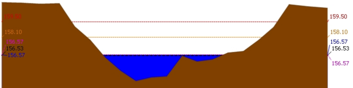
▲ ระดับปัจจุบัน --- ระดับวิกฤติ --- ระดับฝายระวัง ---- เมื่อวาน 7:00 น. - - - - คาดการณ์ล่วงหน้า 1 วัน สถานี 120305T หัวน้ำพุที่ อ.หล่มเก่า จ.เพชรบูรณ์ ระดับน้ำ 156.57 ม.รทก.
