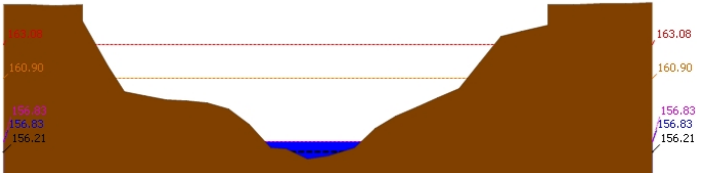
▲ ระดับปัจจุบัน --- ระดับวิกฤติ --- ระดับฝายระวัง ---- เมื่อวาน 7:00 น. - - - - คาดการณ์ล่วงหน้า 1 วัน สถานี 120105T แม่น้ำป่าสักที่บ้านวังมเหสี อ.ท่าอิฐ จ.พิษณุโลก ระดับน้ำ 156.83 ม.รทก.
