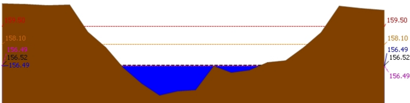
▲ ระดับปัจจุบัน --- ระดับวิกฤติ --- ระดับเฟิาจะวัง ---- เมื่อวาน 7:00 น. - - - - - คาดการณ์ล่วงหน้า 1 วัน สถานี 120305T หัวน้ำพุทที่ อ.หล่มเก่า ต.หล่มเก่า อ.หล่มเก่า จ.เพชรบูรณ์ ระดับน้ำ 156.49 ม.รทก.
