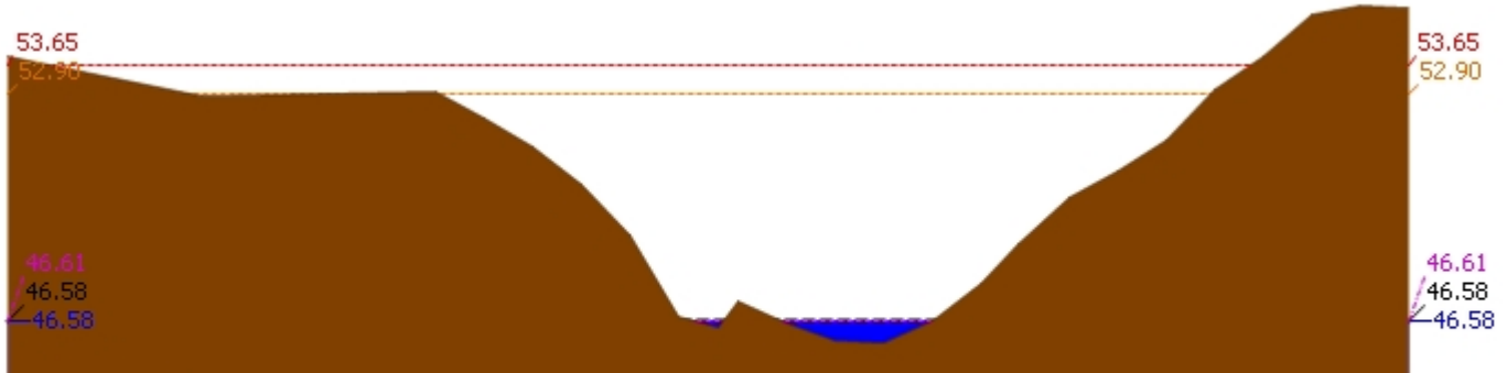
▲ ระดับปัจจุบัน --- ระดับวิกฤติ --- ระดับเฝ้าระวัง ---- เมื่อกวาน 7:00 น. - - - - คาดการณ์ล่วงหน้า 1 วัน สถานี 120113T แม่น้ำป่าสักที่บ้านเขาค้าง ต.คลองกระจิง อ.ศรีเทพ จ.เพชรบูรณ์ ระดับน้ำ 46.58 ม.รทก.
