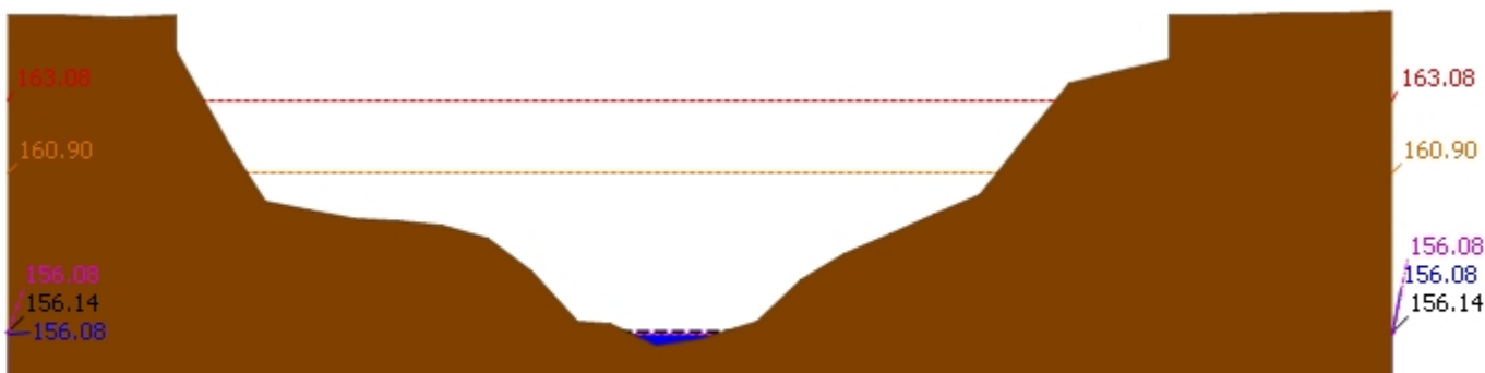
▲ ระดับปัจจุบัน --- ระดับวิกฤติ --- ระดับเฟิาจะวัง ---- เมื่อวาน 7:00 น. - - - - - คาดการณ์ล่วงหน้า 1 วัน สถานี 120105T แม่น้ำป่าสักที่บ้านวังมเสหนือ ต.ทำอิมญ อ.หล่มสัก จ.เพชรบูรณ์ ระดับน้ำ 156.08 ม.รทก.
