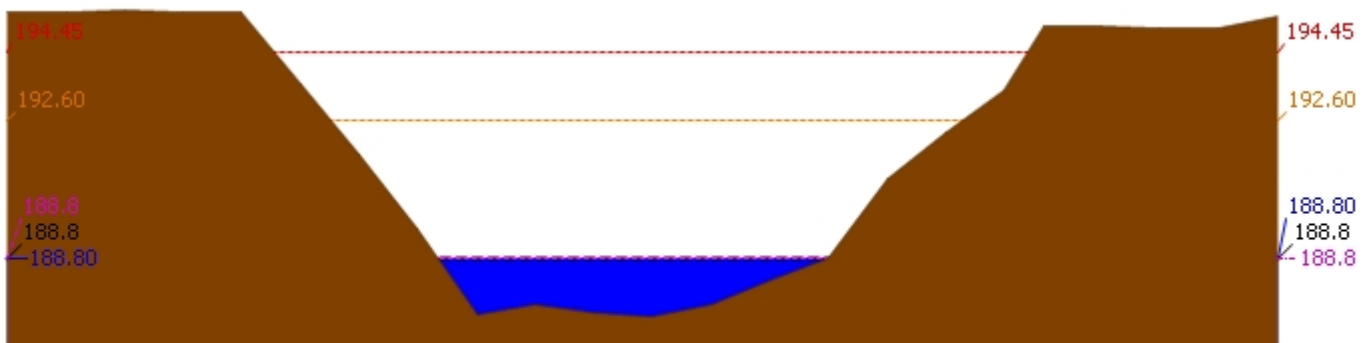
▲ ระดับปัจจุบัน --- ระดับวิกฤติ --- ระดับเฝ้าระวัง ---- เมื่อกวาน 7:00 น. - - - - คาดการณ์ล่วงหน้า 1 วัน สถานี 120901T ห้วยมวกเหล็กที่ อ.มวกเหล็ก ต.มวกเหล็ก อ.มวกเหล็ก จ.สระบุรี ระดับน้ำ 188.80 ม.รทก.
