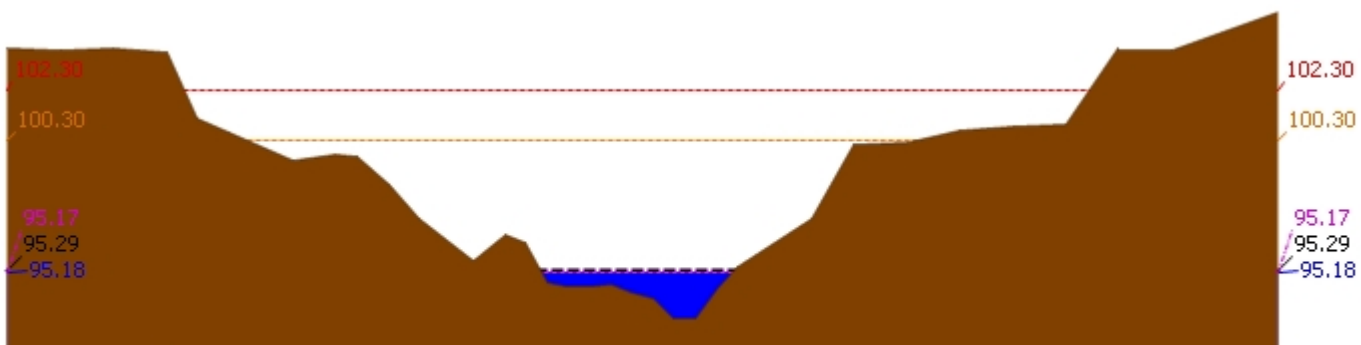
▲ ระดับปัจจุบัน --- ระดับวิกฤติ --- ระดับเฟิาจะวัง ---- เมื่อวาน 7:00 น. - - - - - คาดการณ์ล่วงหน้า 1 วัน สถานี 120112T แม่น้ำป่าสักที่บ้านหนองแหวน ต.วังมะข่อ อ.เมือง จ.เพชรบูรณ์ ระดับน้ำ 95.18 ม.รทก.
