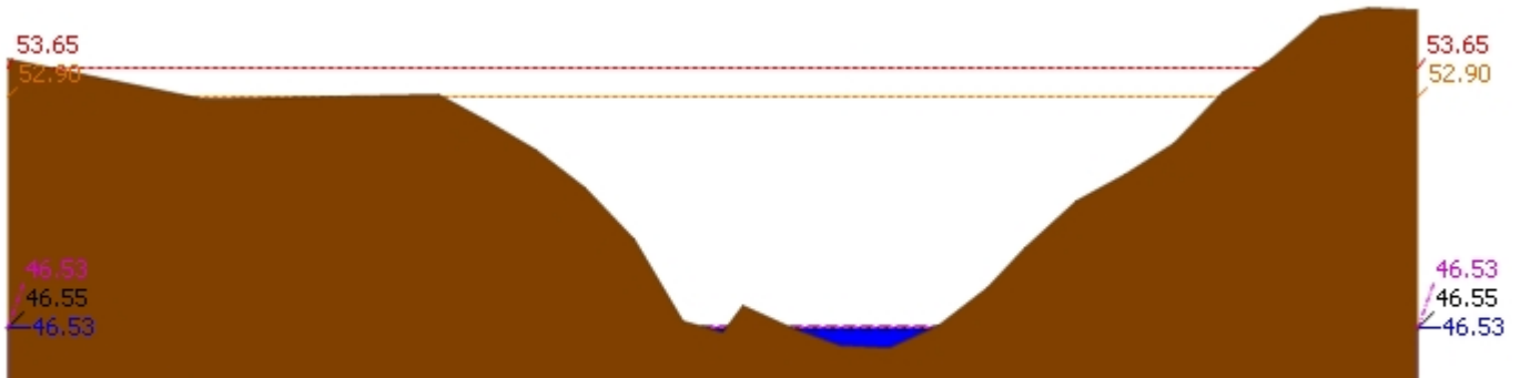
▲ ระดับปัจจุบัน --- ระดับวิกฤติ --- ระดับเฝ้าระวัง ---- เมื่อกาน 7:00 น. - - - - คาดการณ์ล่วงหน้า 1 วัน สถานี 120113T แม่น้ำป่าสักที่บ้านเขาค้าง ต.คลองกระจิง อ.ศรีเทพ จ.เพชรบูรณ์ ระดับน้ำ 46.53 ม.รทก.
