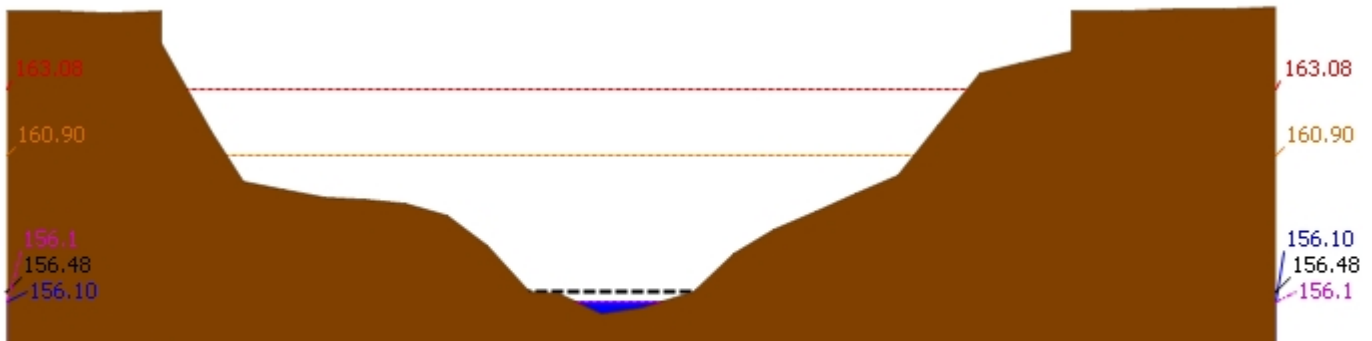
▲ ระดับปัจจุบัน --- ระดับวิกฤติ --- ระดับเฟิาระวัง ---- เมื่อวาน 7:00 น. - - - - คาคการลลวงหน้า 1 วัน สถานี 120105T แม่น้ำป่าสักที่บ้านวังมเสหนือ ต.ทำอญญ อ.หล่มสัก จ.เพชรบูรณ์ ระดับน้ำ 156.10 ม.รทก.
