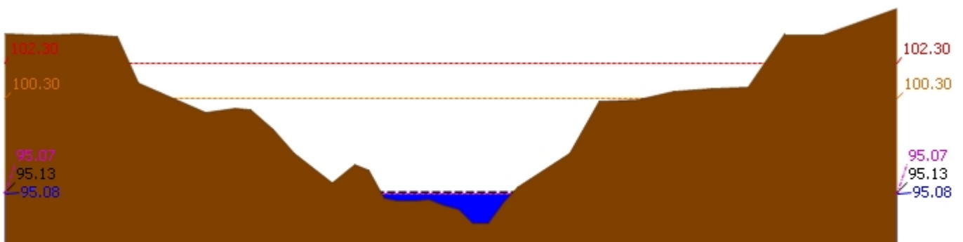
▲ ระดับปัจจุบัน --- ระดับวิกฤติ --- ระดับเฟิาระวัง ---- เมื่อวาน 7:00 น. - - - - คาคการลลวงหน้า 1 วัน สถานี 120112T แม่น้ำป่าสักที่บ้านหนองแหวน ต.วังมะซ่อ อ.เมือง จ.เพชรบูรณ์ ระดับน้ำ 95.08 ม.รทก.
