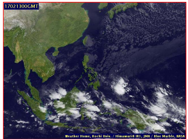
ภาพถ่ายจากดาวเทียม วันที่ ๑๓ ก.พ. ๒๕๖๐ เวลา ๐๗.๐๐ น.
