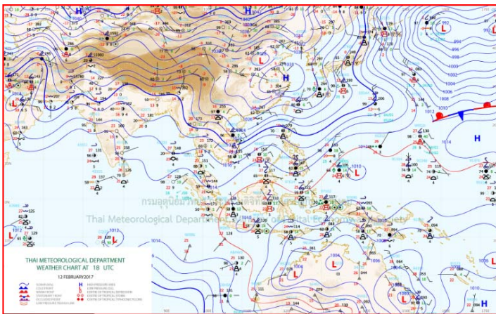
แผนที่อากาศ วันที่ ๑๓ ก.พ. ๒๕๖๐ เวลา ๐๑.๐๐ น.
