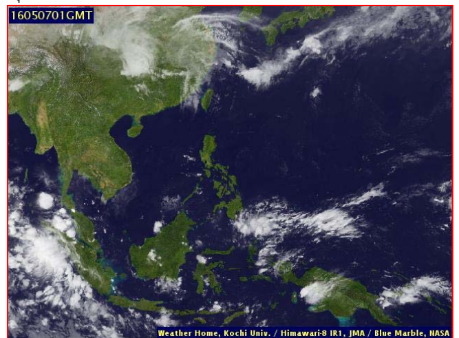
ภาพถ่ายจากดาวเทียม วันที่ ๗ พ.ค. ๒๕๕๙ เวลา ๐๘.๐๐ น.
