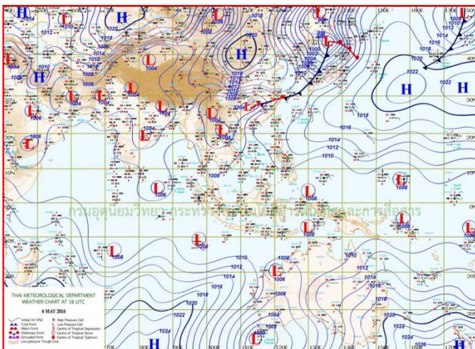
แผนที่อากาศ วันที่ ๗ พ.ค. ๒๕๕๙ เวลา ๐๖.๐๐ น.
