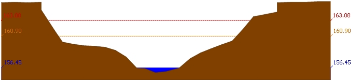
สถานี 120105T แม่น้ำป่าสักที่บ้านวังมเสหนือ ต.ท่าอิฐ อ.หล่มสัก จ.เพชรบูรณ์ ระดับน้ำ 156.45 ม.รทก.
