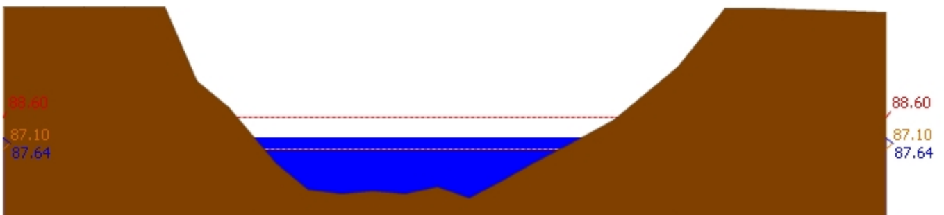
สถานี 120110T แม่น้ำป่าสักที่บ้านวังโบสถ์ ต.วังโบสถ์ อ.หนองไผ่ จ.เพชรบูรณ์ ระดับน้ำ 87.64 ม.รทก.
