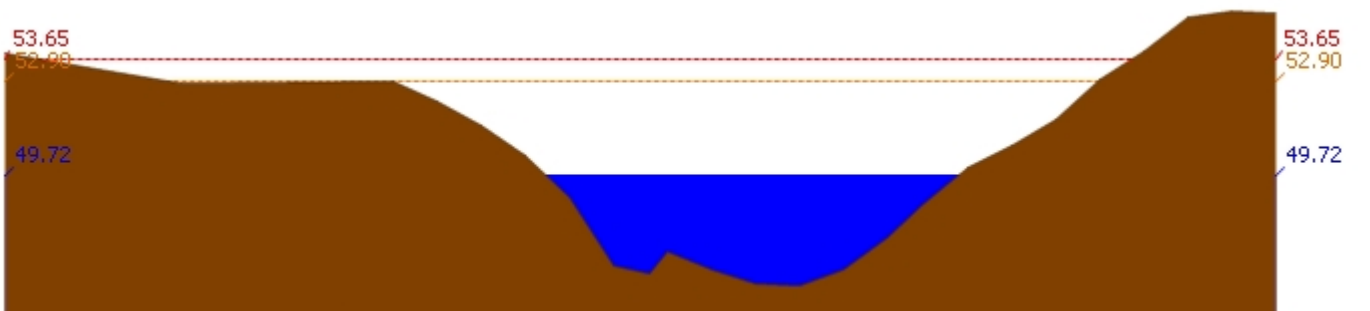
สถานี 120113T แม่น้ำป่าสักที่บ้านเขาค้าง ต.คลองกระจิง อ.ศรีเทพ จ.เพชรบูรณ์ ระดับน้ำ 49.72 ม.รทก.
