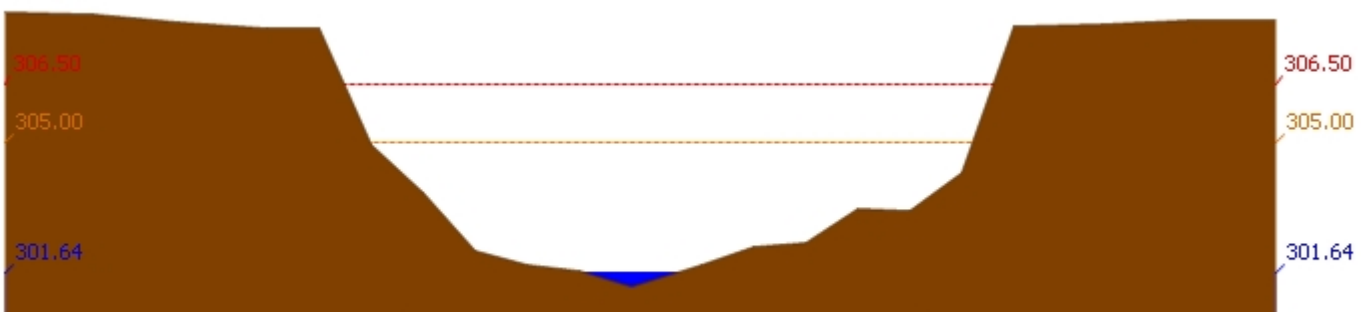
สถานี 120304T ห้วยน้ำพุที่บ้านกกกะบาก ต.โป่ง อ.ด่านซ้าย จ.เลย ระดับน้ำ 301.64 ม.รทก.
