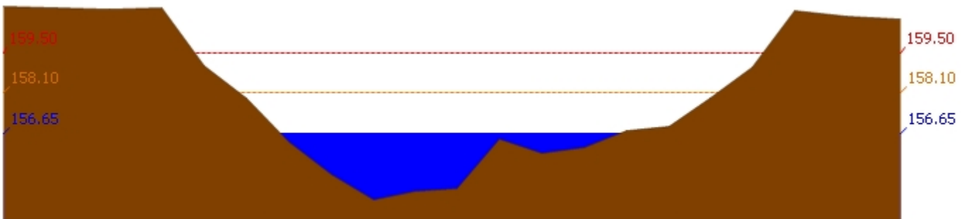
สถานี 120305T หัวขบวนที่ อ.หล่มเก่า ต.หล่มเก่า อ.หล่มเก่า จ.เพชรบูรณ์ ระดับน้ำ 156.65 ม.รทก.
