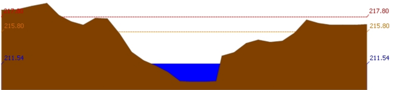
สถานี 120205T แม่น้ำป่าสักที่บ้านอู่กระทัด ต.ศิลา อ.หล่มเก่า จ.เพชรบูรณ์ ระดับน้ำ 211.54 ม.รทก.
