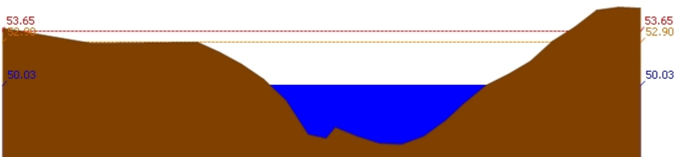
สถานี 120113T แม่น้ำป่าสักที่บ้านเขาค้าง ต.คลองกระจิง อ.ศรีเทพ จ.เพชรบูรณ์ ระดับน้ำ 50.03 ม.รทก.
