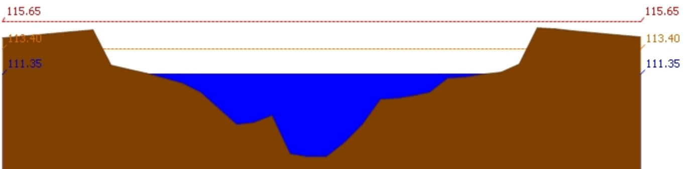
สถานี 120107T แม่น้ำป่าสักที่ อ.เมืองเพชรบูรณ์ ต.นาป่า อ.เมือง จ.เพชรบูรณ์ ระดับน้ำ 111.35 ม.รทก.
