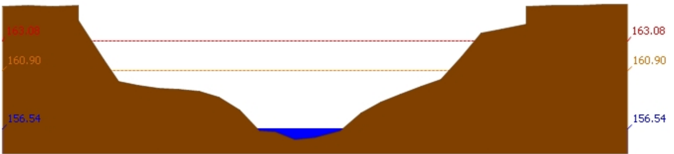
สถานี 120105T แม่น้ำป่าสักที่บ้านวังมเสหนือ ต.ทำอัญญ อ.หล่มสัก จ.เพชรบูรณ์ ระดับน้ำ 156.54 ม.รทก.
