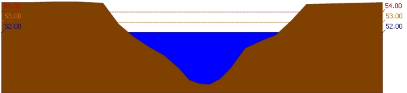
สถานี 120702T ลำสนธิที่บ้านท่าช้าง ต.หนองขาหย่าง อ.ชัยบาดาล จ.ลพบุรี ระดับน้ำ 52.00 ม.รทก.
