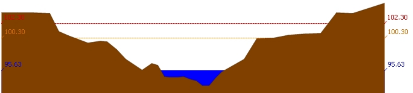
สถานี 120112T แม่น้ำป่าสักที่บ้านหนองแหวน ต.วังมะข่อ อ.เมือง จ.เพชรบูรณ์ ระดับน้ำ 95.63 ม.รทก.
