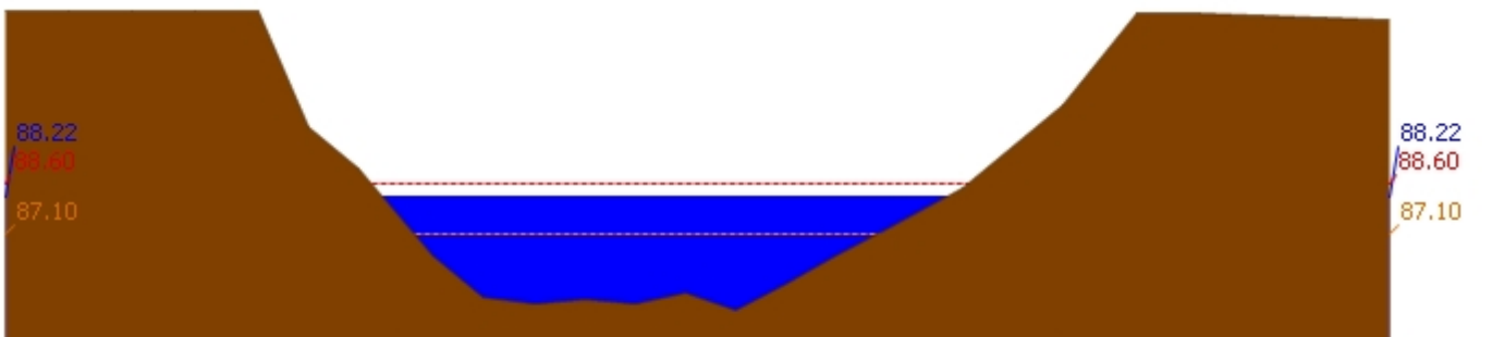
สถานี 120110T แม่น้ำป่าสักที่บ้านวังโบสถ์ ต.วังโบสถ์ อ.หนองไผ่ จ.เพชรบูรณ์ ระดับน้ำ 88.22 ม.รทก.
