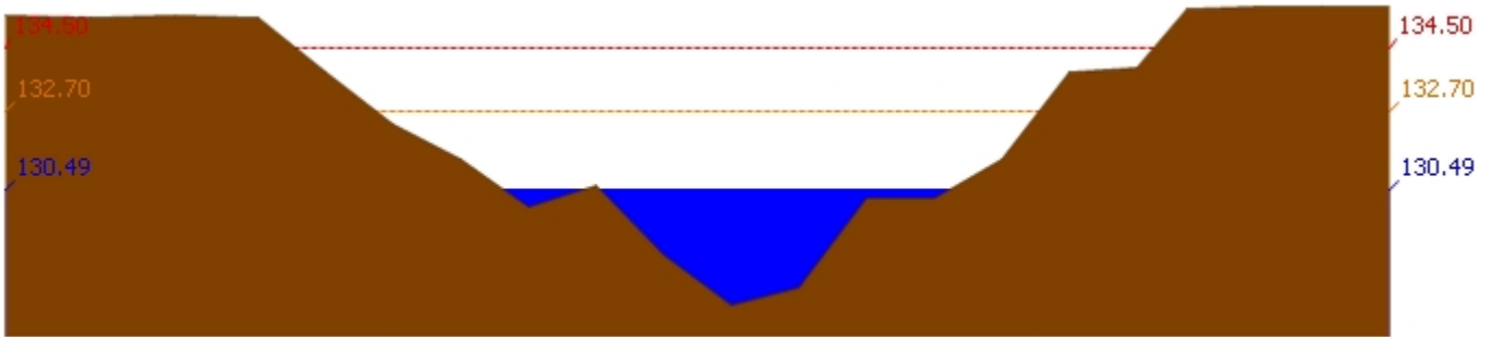
สถานี 120111T แม่น้ำป่าสักที่บ้านจางวาง ต.ลานบัว อ.หล่มสัก จ.เพชรบูรณ์ ระดับน้ำ 130.49 ม.รทก.
