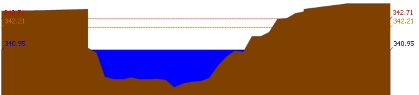
สถานี 070304T น้ำแม่สอยที่บ้านหนองกอก ต.แม่สุก อ.แจ้ห่ม จ.ลำปาง ระดับน้ำ 340.95 ม.รทก.
