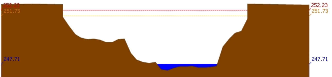
สถานี 070403T น้ำแม่ตุ๋ยที่บ้านแค้ ต.บ้านเป้า อ.เมืองลำปาง จ.ลำปาง ระดับน้ำ 247.71 ม.รทก.
