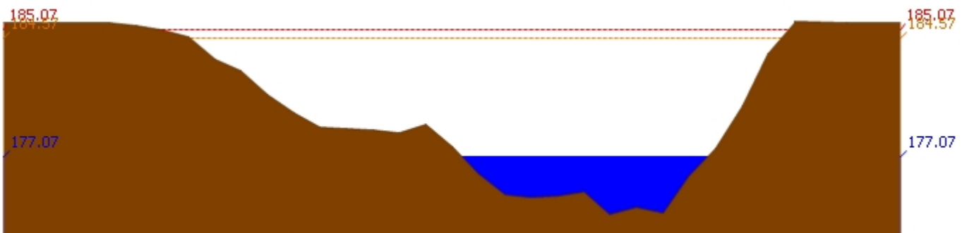
สถานี 070116T แม่น้ำวังที่บ้านแม่เตี๊ยะ ต.แม่ถอด อ.เถิน จ.ลำปาง ระดับน้ำ 177.07 ม.รทก.
