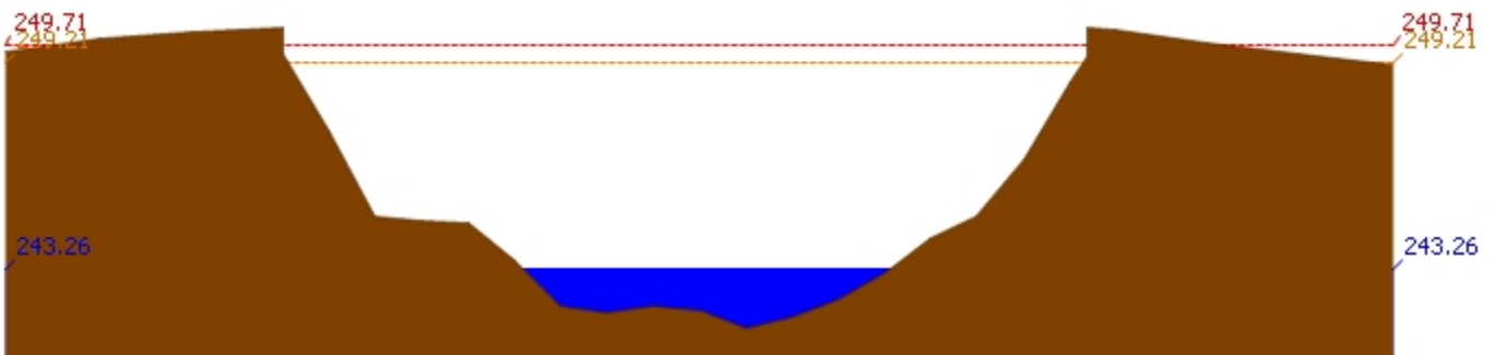
สถานี 070112T แม่น้ำวังที่บ้านบุญนาค ต.บุญนาคพัฒนา อ.เมืองลำปาง จ.ลำปาง ระดับน้ำ 243.26 ม.รทก.
