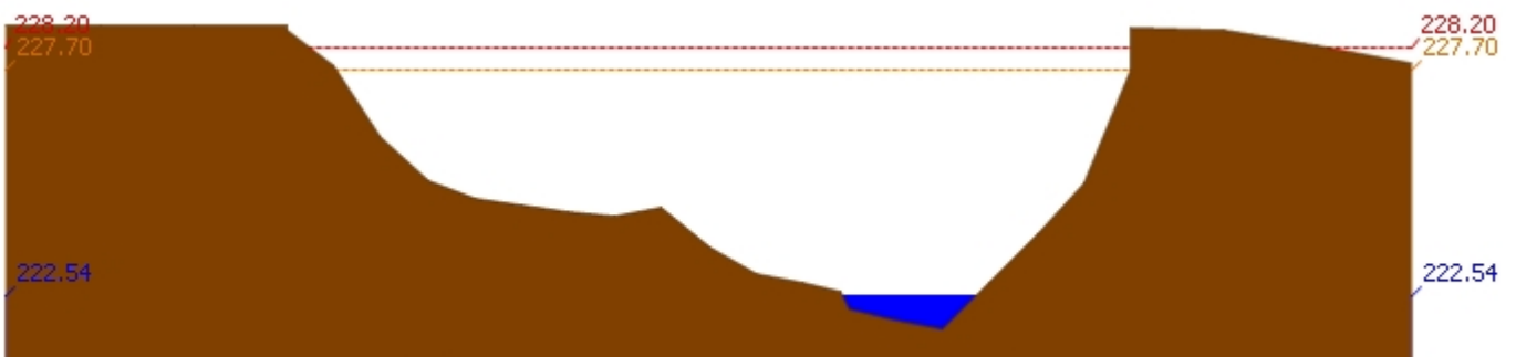
สถานี 070703T น้ำแม่ตำที่บ้านนาบอน ต.ทุ่งงาม อ.เสริมงาม จ.ลำปาง ระดับน้ำ 222.54 ม.รทก.
