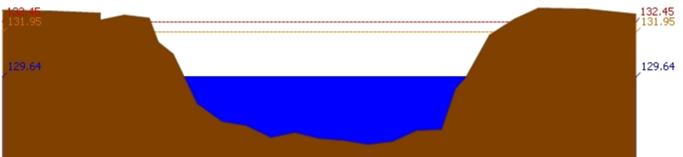
สถานี 070118T แม่น้ำวังที่บ้านแม่สลิด ต.แม่สลิด อ.บ้านตาก จ.ตาก ระดับน้ำ 129.64 ม.รทก.
