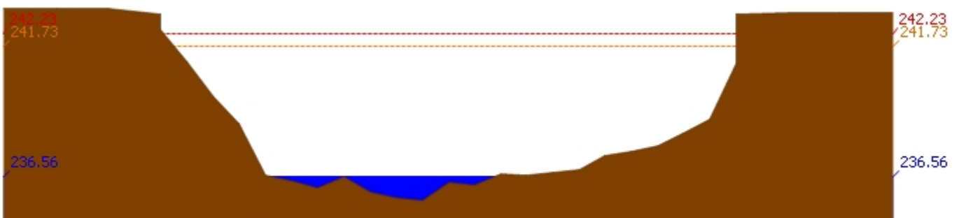
สถานี 070114T แม่น้ำวังที่บ้านปงชัย ต.บ้านเสด็จ อ.เมืองลำปาง จ.ลำปาง ระดับน้ำ 236.56 ม.รทก.
