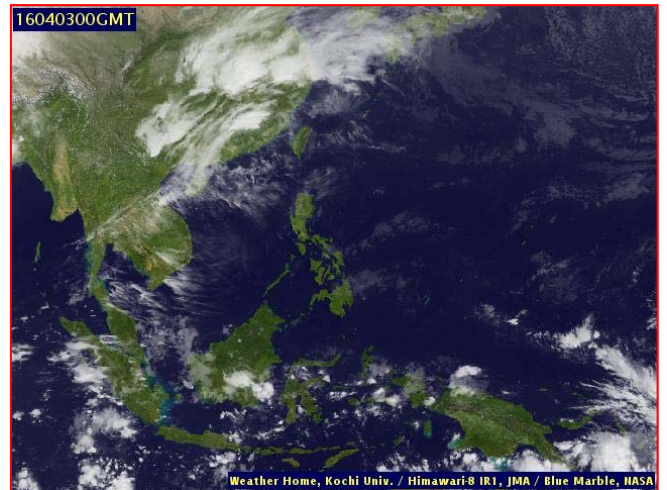
ภาพถ่ายจากดาวเทียม วันที่ ๓ เม.ย. ๒๕๕๙ เวลา ๐๖.๐๐ น.
