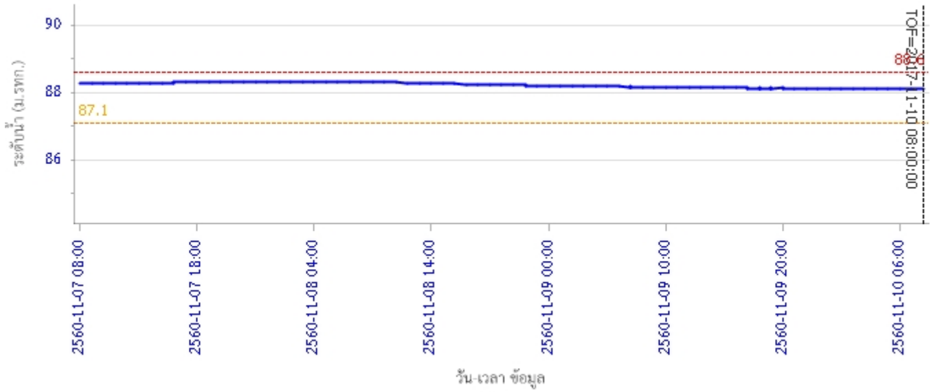
ผลการคำนวณระดับน้ำ สถานี 120304T ห้วยน้ำพุงที่บ้านกกกะบาก ต.โป่ง อ.ด่านซ้าย จ.เลย
