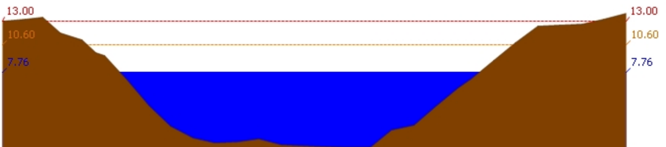
สถานี 120106T แม่น้ำป่าสักที่ อ.เสนาห์ ต.ศาลาวิไทย อ.เสนาห์ จ.สระบุรี ระดับน้ำ 7.76 ม.รทก.
