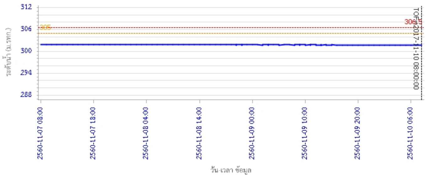
ผลการคำนวณระดับน้ำ สถานี 120304T ห้วยน้ำพุงที่บ้านกกกะบาก ต.โป่ง อ.ด่านซ้าย จ.เลย
