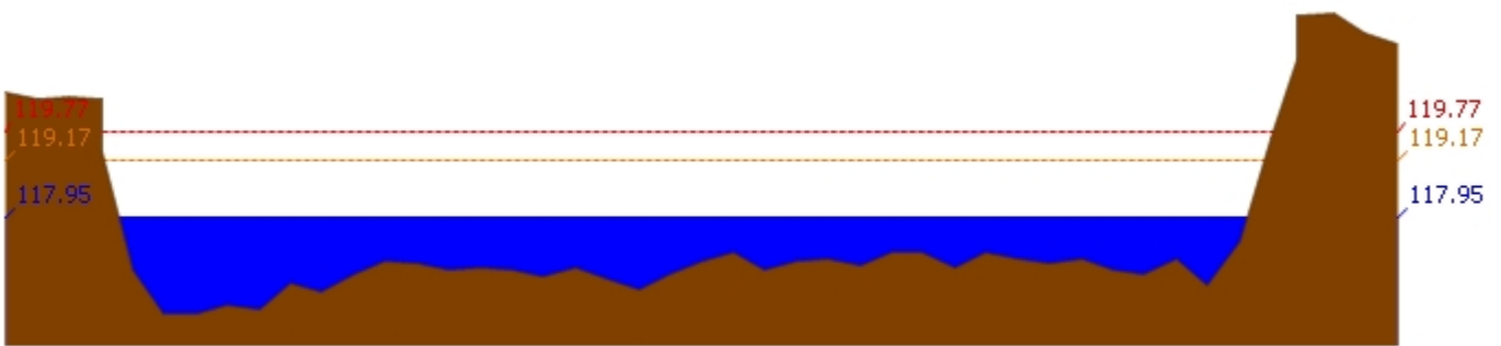
สถานี 060111T แม่น้ำปิงที่บ้านปากร่องห้วยจี่ ต.ตากออก อ.บ้านตาก จ.ตาก ระดับน้ำ 117.95 ม.รทก.
