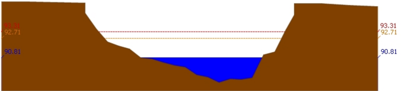
สถานี 061901T คลองแม่ระกาที่บ้านวังชะโอน ต.ท่าไม้ อ.พรานกระต่าย จ.กำแพงเพชร ระดับน้ำ 90.81 ม.รทก.
