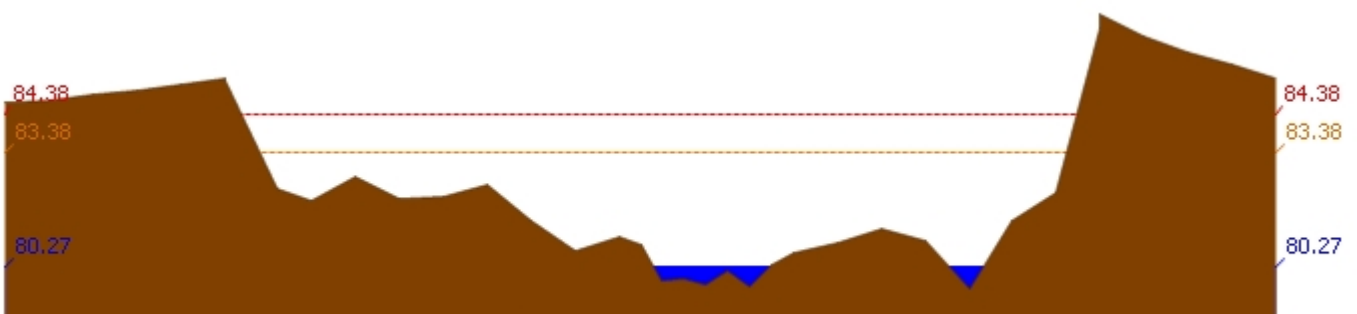
สถานี 062001T คลองสวนหมากที่บ้านน้ำไทรง ต.ท่าขุนราม อ.เมือง จ.กำแพงเพชร ระดับน้ำ 80.27 ม.รทก.
