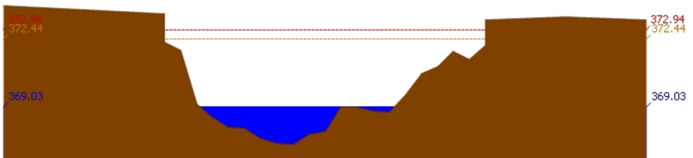
สถานี 060109T แม่น้ำปิงที่บ้านสบอ้อ ต.แม่ทะ อ.เชียงดาว จ.เชียงใหม่ ระดับน้ำ 369.03 ม.รทก.
