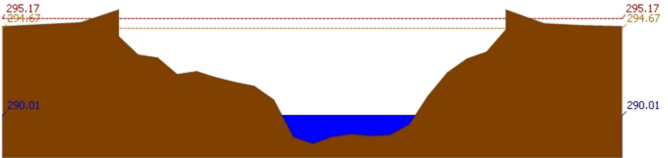
สถานี 060709T น้ำแม่กวังที่ลำพูน ต.เวียงของ อ.เมือง จ.ลำพูน ระดับน้ำ 290.01 ม.รทก.
