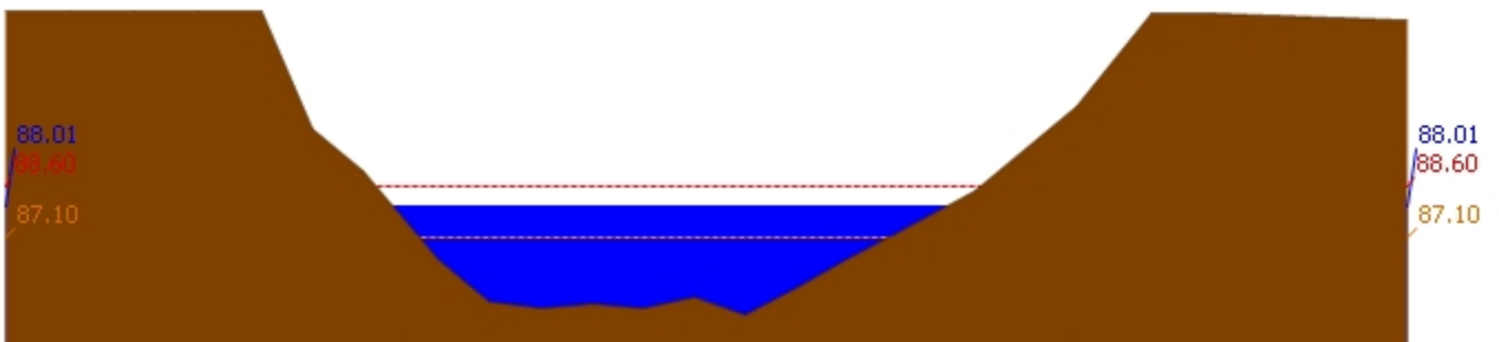
สถานี 120110T แม่น้ำป่าสักที่บ้านวังโบสถ์ ต.วังโบสถ์ อ.หนองไผ่ จ.เพชรบูรณ์ ระดับน้ำ 88.01 ม.รทก.
