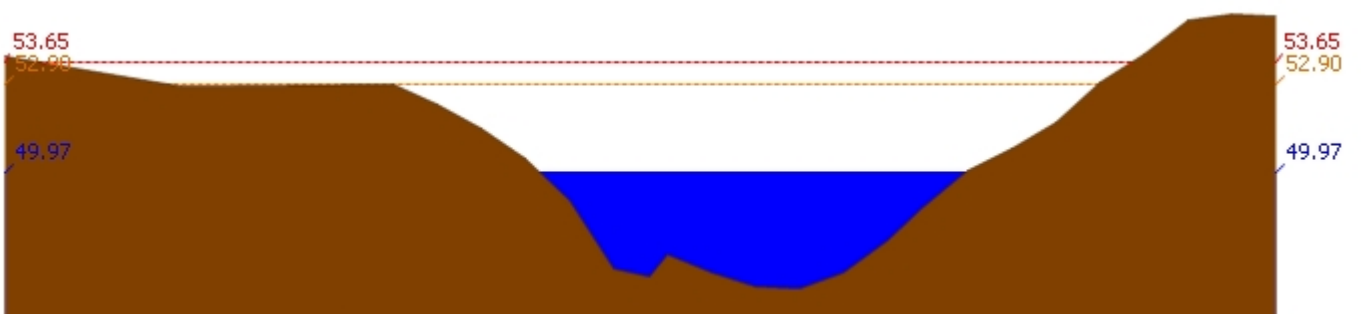
สถานี 120113T แม่น้ำป่าสักที่บ้านเขาค้าง ต.คลองกระจิง อ.ศรีเทพ จ.เพชรบูรณ์ ระดับน้ำ 49.97 ม.รทก.
