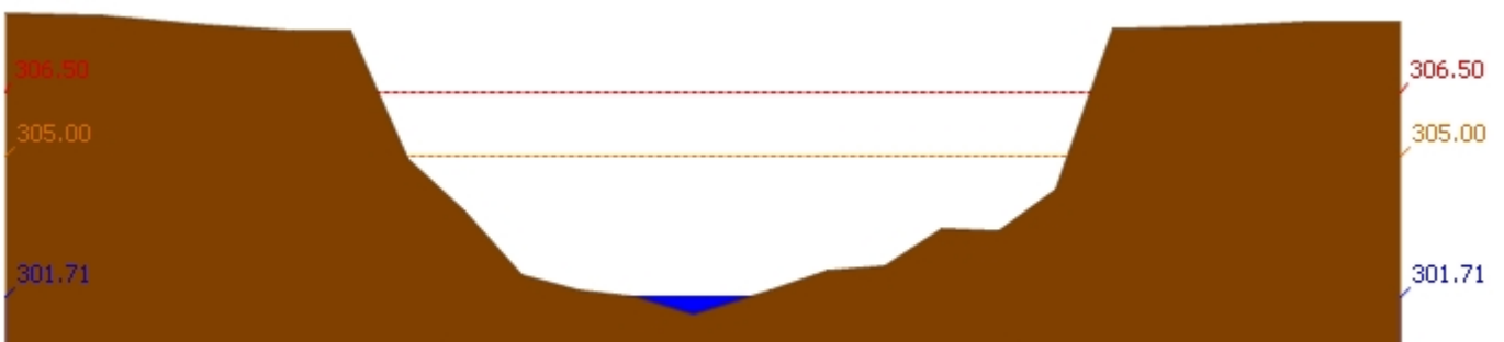
สถานี 120304T ห้วยน้ำพุที่บ้านกกกะบาก ต.โป่ง อ.ด่านซ้าย จ.เลย ระดับน้ำ 301.71 ม.รทก.
