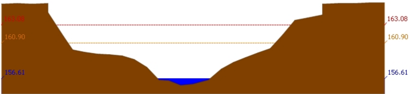
สถานี 120105T แม่น้ำป่าสักที่บ้านวังมเสหนือ ต.ท่าอิบุญ อ.หล่มสัก จ.เพชรบูรณ์ ระดับน้ำ 156.61 ม.รทก.
