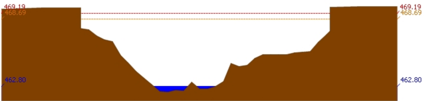
สถานี 060905T น้ำแม่ลี้ที่อำเภอลี้ ต.ลี้ อ.ลี้ จ.ลำพูน ระดับน้ำ 462.80 ม.รทก.
