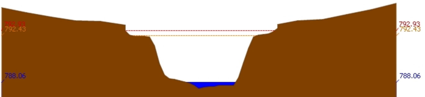
สถานี 061503T น้ำแม่ต้นที่บ้านคอย ต.ยางเปียง อ.อมก๋อย จ.เชียงใหม่ ระดับน้ำ 788.06 ม.รทก.
