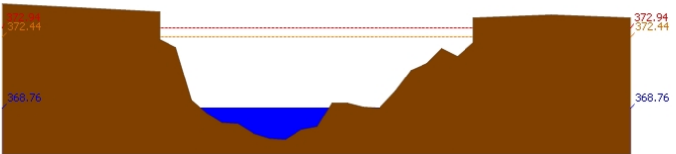
สถานี 060109T แม่น้ำปิงที่บ้านสบอ้อ ต.แม่ระ อ.เชียงดาว จ.เชียงใหม่ ระดับน้ำ 368.76 ม.รทก.
