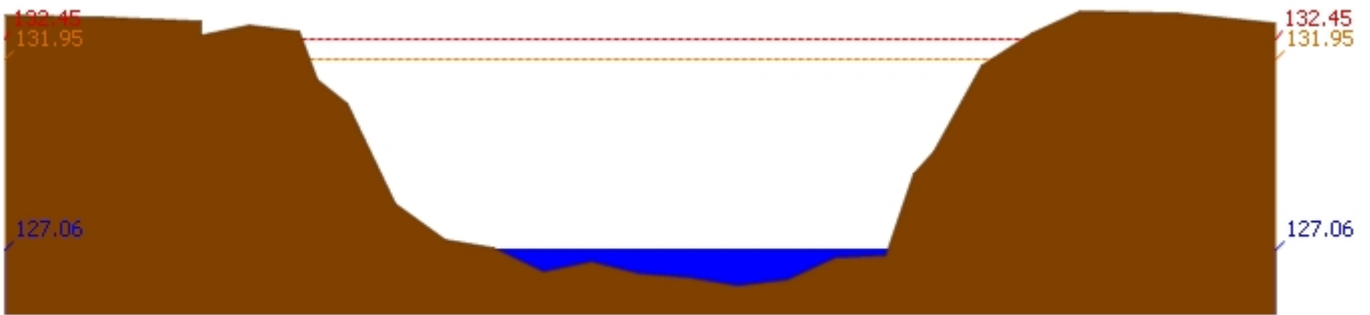
สถานี 070118T แม่น้ำวังที่บ้านแม่สลิด ต.แม่สลิด อ.บ้านตาก จ.ตาก ระดับน้ำ 127.06 ม.รทก.
