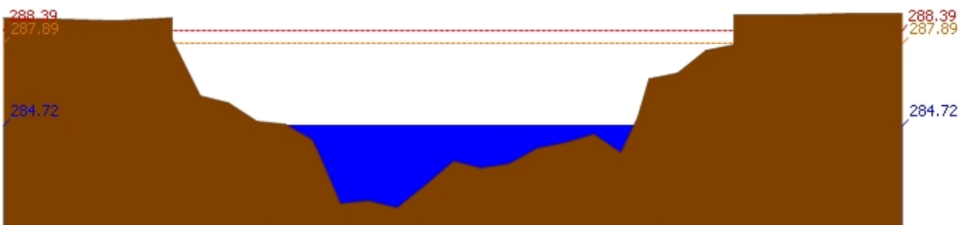
สถานี 070111T แม่น้ำวังที่บ้านโป่งชัย ต.บ้านเสา อ.แจ้ห่ม จ.ลำปาง ระดับน้ำ 284.72 ม.รทก.
