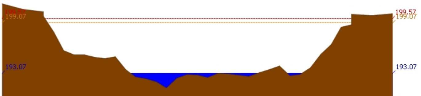
สถานี 070115T น้ำแม่วังที่บ้านอ้อ ต.แม่แก้ว อ.สบปราบ จ.ลำปาง ระดับน้ำ 193.07 ม.รทก.
