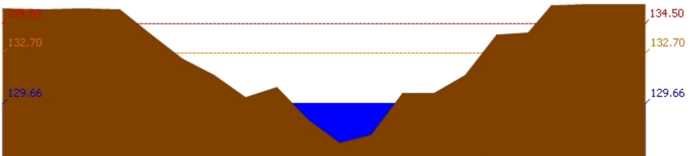
สถานี 120111T แม่น้ำป่าสักที่บ้านจางวาง ต.ลานบัว อ.หล่มสัก จ.เพชรบูรณ์ ระดับน้ำ 129.66 ม.รทก.
