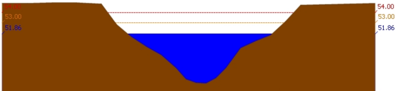
สถานี 120702T ลำสนธิที่บ้านท่าช้าง ต.หนองขาหย่าง อ.ชัยบาดาล จ.ลพบุรี ระดับน้ำ 51.86 ม.รทก.
