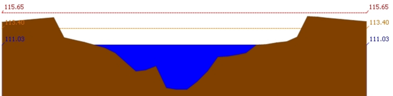
สถานี 120107T แม่น้ำป่าสักที่ อ.เมืองเพชรบูรณ์ ต.นาป่า อ.เมือง จ.เพชรบูรณ์ ระดับน้ำ 111.03 ม.รทก.
