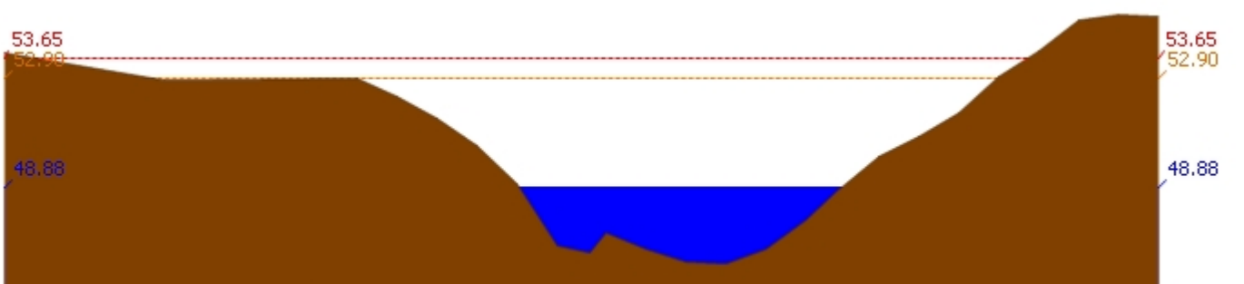
สถานี 120113T แม่น้ำป่าสักที่บ้านเขาค้าง ต.คลองกระจิง อ.ศรีเทพ จ.เพชรบูรณ์ ระดับน้ำ 48.88 ม.รทก.
