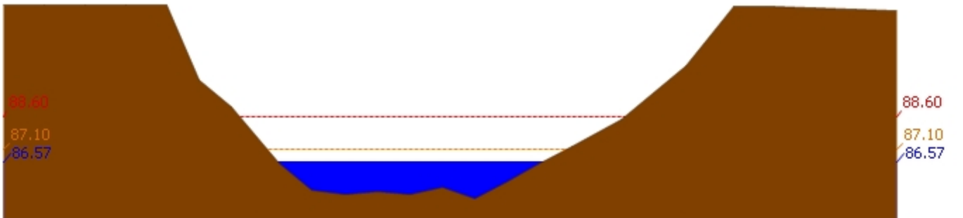
สถานี 120110T แม่น้ำป่าสักที่บ้านวังโบสถ์ ต.วังโบสถ์ อ.หนองไผ่ จ.เพชรบูรณ์ ระดับน้ำ 86.57 ม.รทก.
