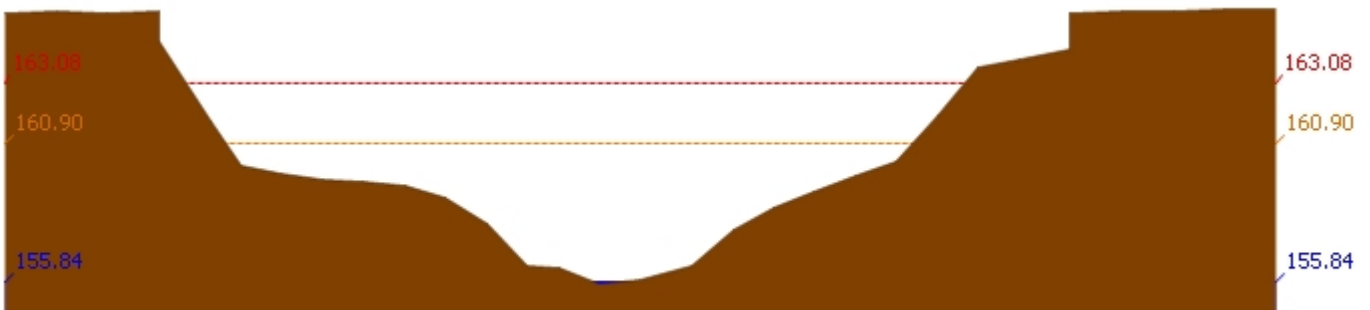
สถานี 120105T แม่น้ำป่าสักที่บ้านวังมเหนื่อ ต.ทำอิบุญ อ.หล่มสัก จ.เพชรบูรณ์ ระดับน้ำ 155.84 ม.รทก.
