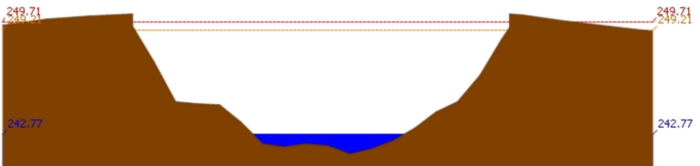
สถานี 070112T แม่น้ำวังที่บ้านบุญนาคน ต.บุญนาคนพัฒนา อ.เมืองลำปาง จ.ลำปาง ระดับน้ำ 242.77 ม.รทก.
