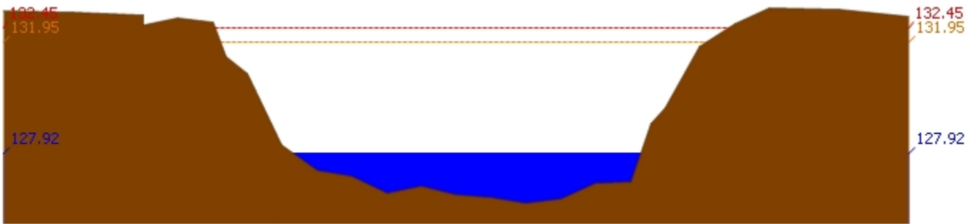
สถานี 070118T แม่น้ำวังที่บ้านแม่สลิด ต.แม่สลิด อ.บ้านตาก จ.ตาก ระดับน้ำ 127.92 ม.รทก.
