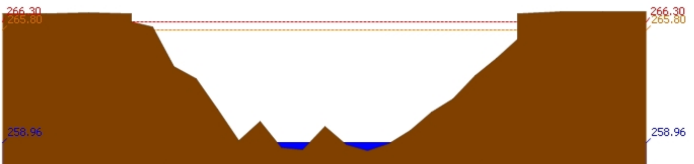
สถานี 070604T น้ำแม่จางที่บ้านสุโขทัยมงคล ต.หัวเสือ อ.แม่ทะ จ.ลำปาง ระดับน้ำ 258.96 ม.รทก.
