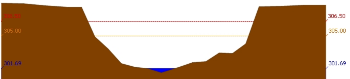
สถานี 120304T หัวน้ำพุที่บ้านกกกะบาก ต.โป่ง อ.ด่านซ้าย จ.เลย ระดับน้ำ 301.69 ม.รทก.
