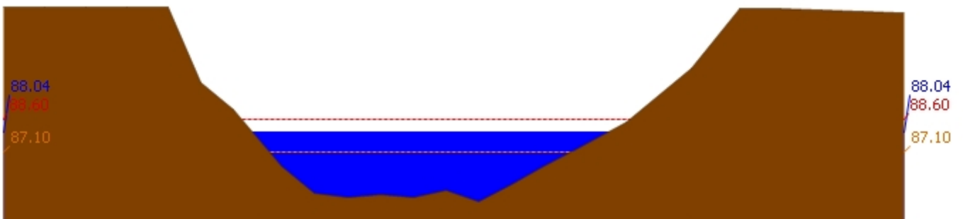
สถานี 120110T แม่น้ำป่าสักที่บ้านวังโบสถ์ ต.วังโบสถ์ อ.หนองไผ่ จ.เพชรบูรณ์ ระดับน้ำ 88.04 ม.รทก.
