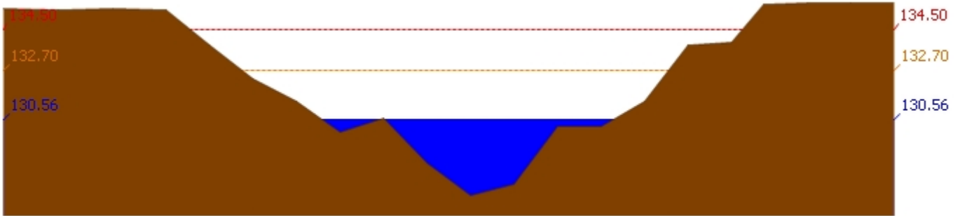
สถานี 120111T แม่น้ำป่าสักที่บ้านจางวาง ต.ลานบัว อ.หล่มสัก จ.เพชรบูรณ์ ระดับน้ำ 130.56 ม.รทก.
