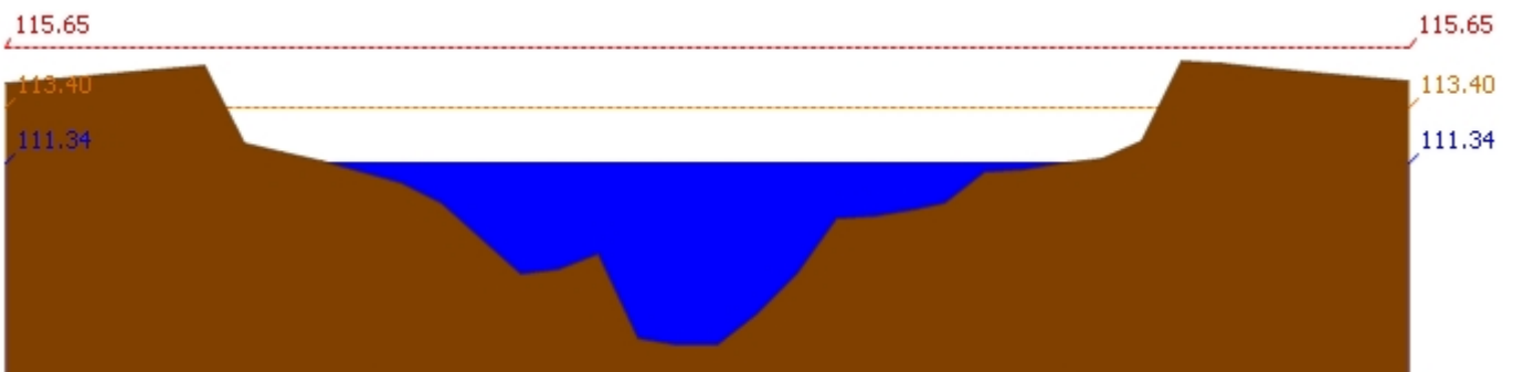
สถานี 120107T แม่น้ำป่าสักที่ อ.เมืองเพชรบูรณ์ ต.นาป่า อ.เมือง จ.เพชรบูรณ์ ระดับน้ำ 111.34 ม.รทก.
