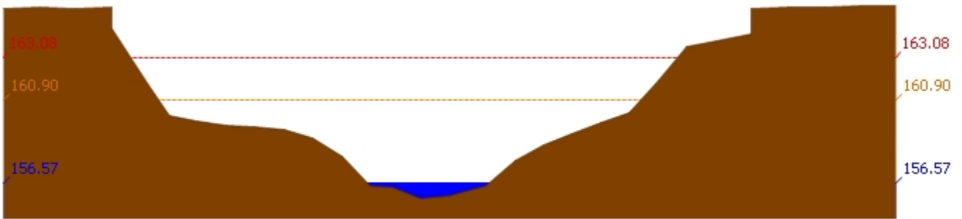
สถานี 120105T แม่น้ำป่าสักที่บ้านวังมเสหนือ ต.ท่าอิฐ อ.หล่มสัก จ.เพชรบูรณ์ ระดับน้ำ 156.57 ม.รทก.
