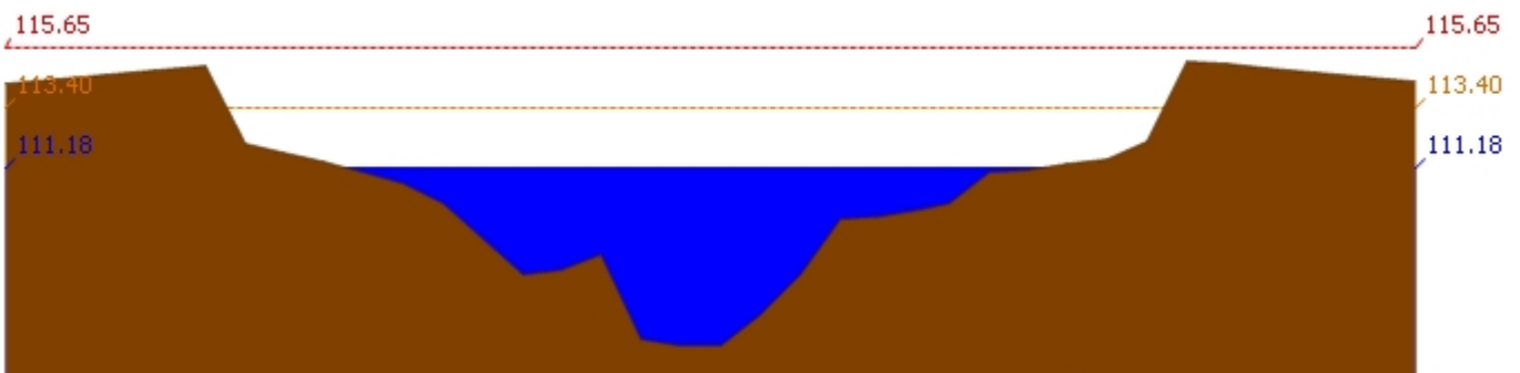
สถานี 120107T แม่น้ำป่าสักที่ อ.เมืองเพชรบูรณ์ ต.นาป่า อ.เมือง จ.เพชรบูรณ์ ระดับน้ำ 111.18 ม.รทก.
