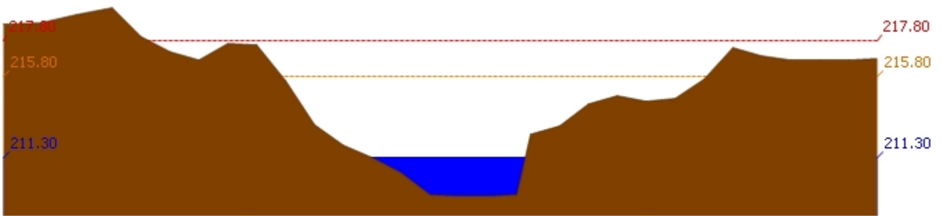
สถานี 120205T แม่น้ำป่าสักที่บ้านอู่กระทัด ต.ศิลา อ.หล่มเก่า จ.เพชรบูรณ์ ระดับน้ำ 211.30 ม.รทก.
