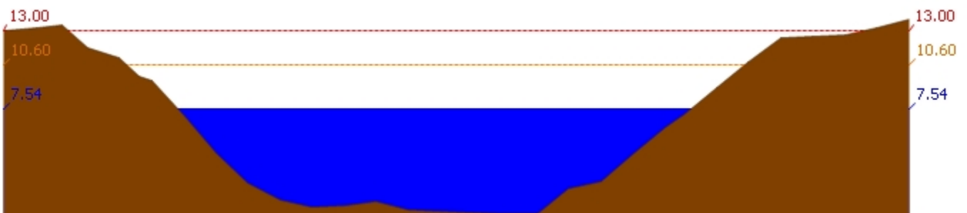
สถานี 120106T แม่น้ำป่าสักที่ อ.เสนาห์ ต.ศาลาวิไทย อ.เสนาห์ จ.สระบุรี ระดับน้ำ 7.54 ม.รทก.
