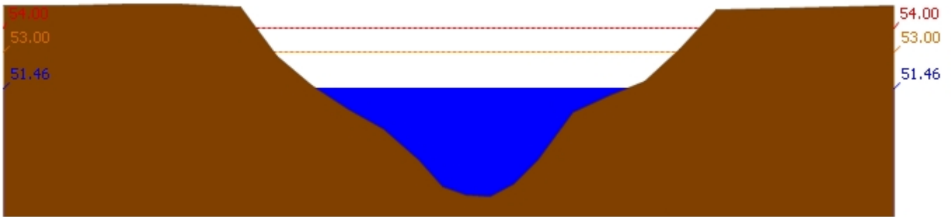
สถานี 120702T ลำสนธิที่บ้านท่าช้าง ต.หนองขาหย่าง อ.ชัยบาดาล จ.ลพบุรี ระดับน้ำ 51.46 ม.รทก.
