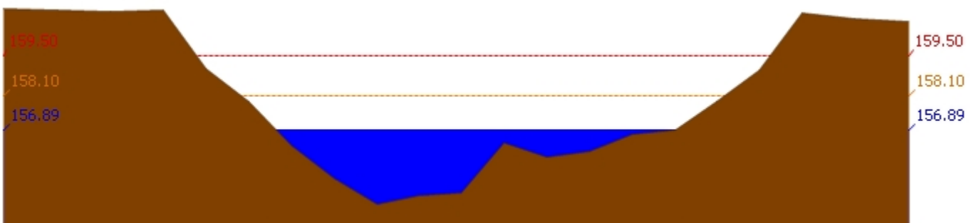
สถานี 120305T หัวน้ำพุที่ อ.หล่มเก่า ต.หล่มเก่า อ.หล่มเก่า จ.เพชรบูรณ์ ระดับน้ำ 156.89 ม.รทก.
