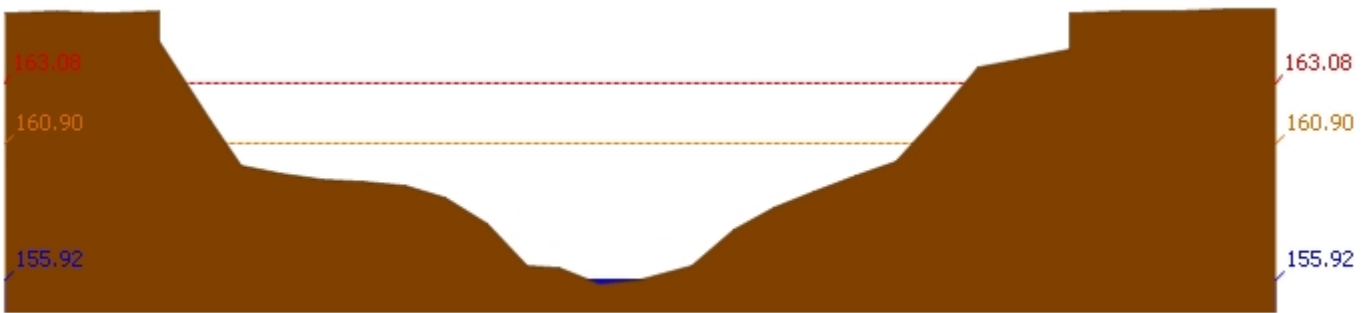
สถานี 120105T แม่น้ำป่าสักที่บ้านวังมเสหนือ ต.ท่าอิบุญ อ.หล่มสัก จ.เพชรบูรณ์ ระดับน้ำ 155.92 ม.รทก.
