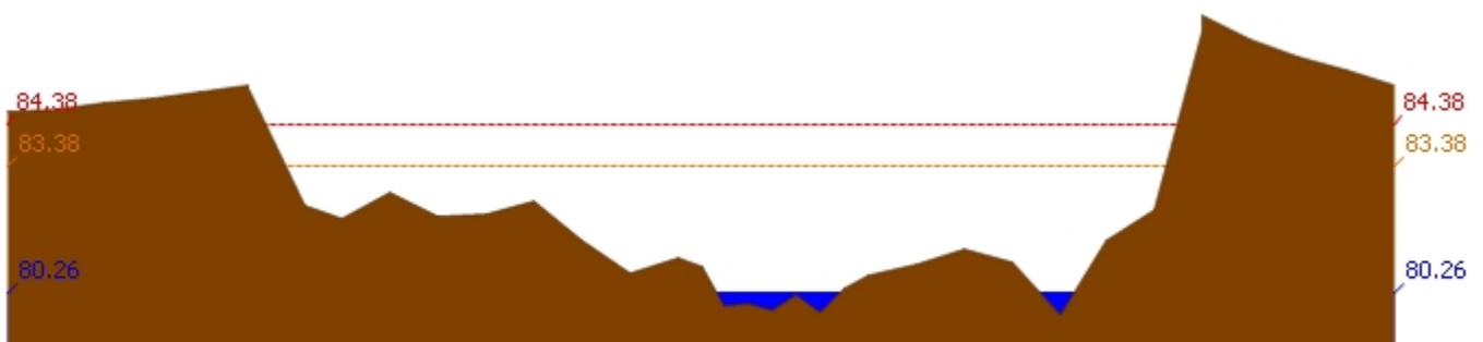
สถานี 062001T คลองสวนหมากที่บ้านน้ำไทรง ต.ท่าขุนราม อ.เมือง จ.กำแพงเพชร ระดับน้ำ 80.26 ม.รทก.
