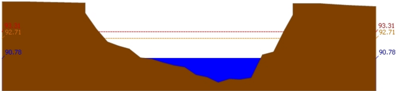
สถานี 061901T คลองแม่ระกาที่บ้านวังชะโอน ต.ท่าไม้ อ.พรานกระต่าย จ.กำแพงเพชร ระดับน้ำ 90.78 ม.รทก.
