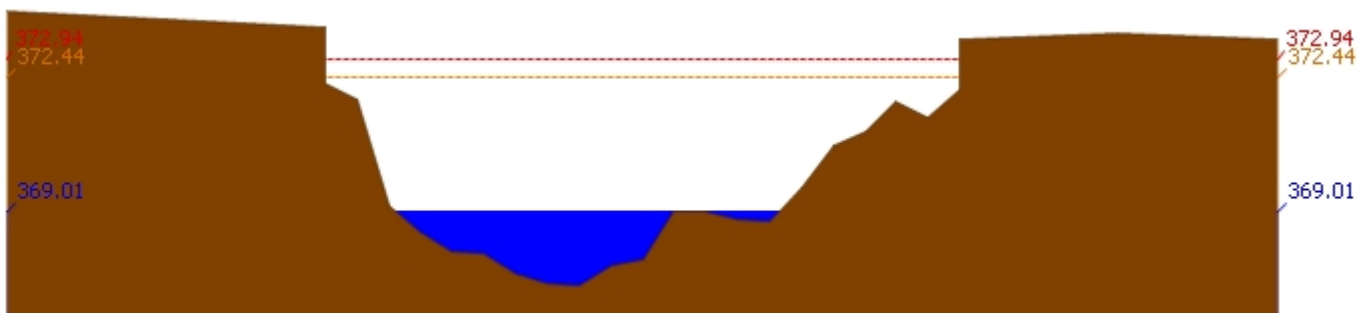
สถานี 060109T แม่น้ำปิงที่บ้านสบอ้อ ต.แม่ทะ อ.เชียงดาว จ.เชียงใหม่ ระดับน้ำ 369.01 ม.รทก.
