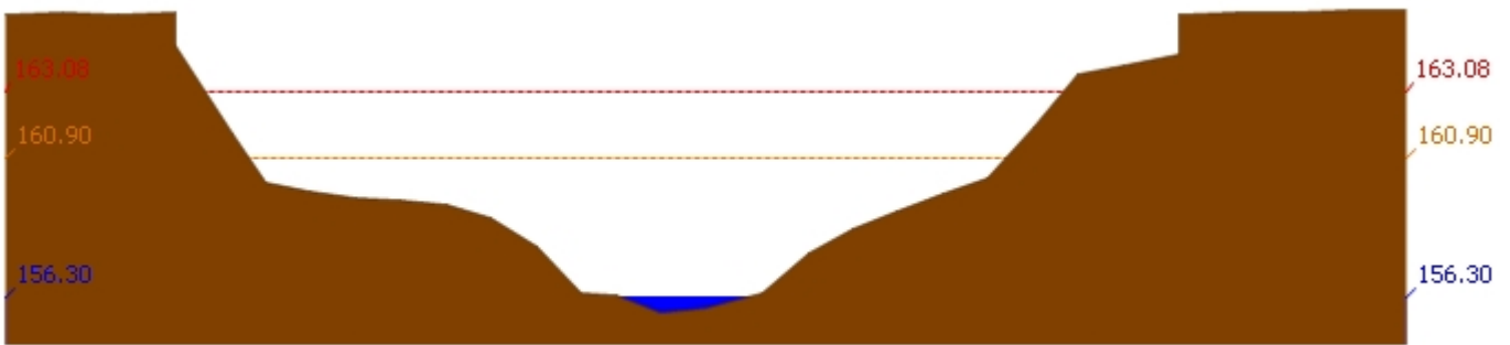
สถานี 120105T แม่น้ำป่าสักที่บ้านวังมเสหนือ ต.ทำอิบุญ อ.หล่มสัก จ.เพชรบูรณ์ ระดับน้ำ 156.30 ม.รทก.
