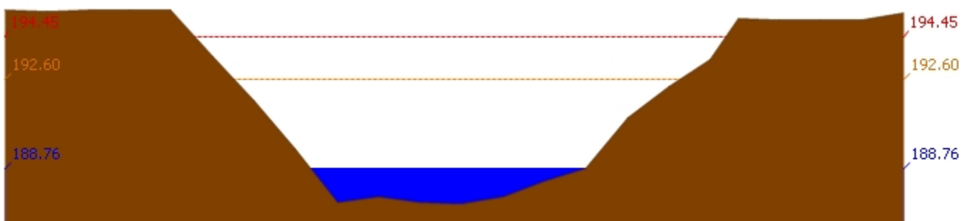
สถานี 120901T ห้วยมวกเหล็กที่ อ.มวกเหล็ก ต.มวกเหล็ก อ.มวกเหล็ก จ.สระบุรี ระดับน้ำ 188.76 ม.รทก.
