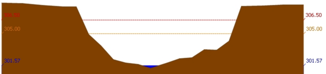
สถานี 120304T ห้วยน้ำพุที่บ้านกกกะบาก ต.โป่ง อ.ด่านซ้าย จ.เลย ระดับน้ำ 301.57 ม.รทก.
