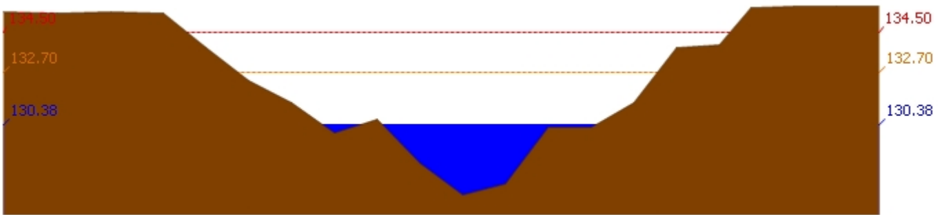
สถานี 120111T แม่น้ำป่าสักที่บ้านจางวาง ต.ลานบัว อ.หล่มสัก จ.เพชรบูรณ์ ระดับน้ำ 130.38 ม.รทก.
