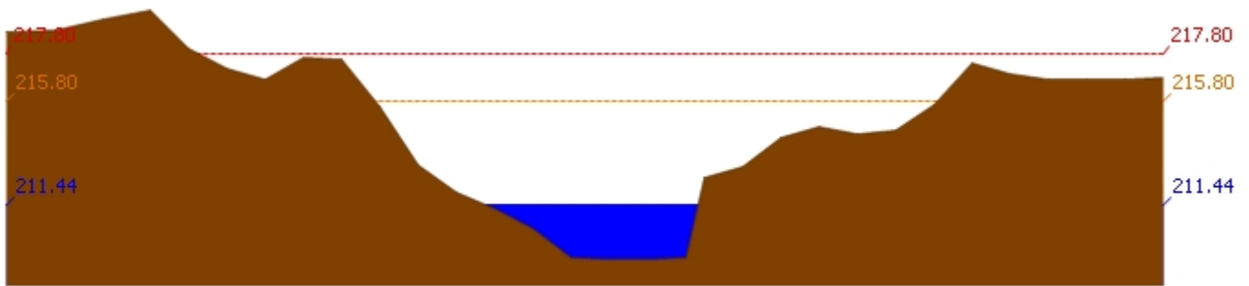
สถานี 120205T แม่น้ำป่าสักที่บ้านอู่กระทัด ต.ศิลา อ.หล่มเก่า จ.เพชรบูรณ์ ระดับน้ำ 211.44 ม.รทก.
