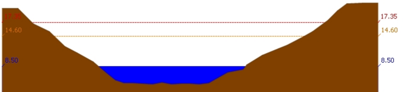
สถานี 120109T แม่น้ำป่าสักที่ อ.แก่งคอย ต.แก่งคอย อ.แก่งคอย จ.สระบุรี ระดับน้ำ 8.50 ม.รทก.
