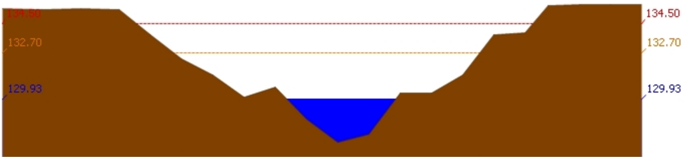
สถานี 120111T แม่น้ำป่าสักที่บ้านจางวาง ต.ลานบัว อ.หล่มสัก จ.เพชรบูรณ์ ระดับน้ำ 129.93 ม.รทก.
