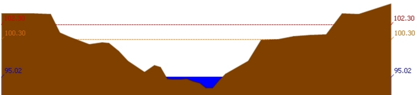
สถานี 120112T แม่น้ำป่าสักที่บ้านหนองแหวน ต.วังมะข่อ อ.เมือง จ.เพชรบูรณ์ ระดับน้ำ 95.02 ม.รทก.
