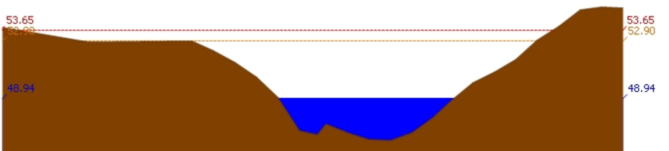
สถานี 120113T แม่น้ำป่าสักที่บ้านเขาค้าง ต.คลองกระจิง อ.ศรีเทพ จ.เพชรบูรณ์ ระดับน้ำ 48.94 ม.รทก.
