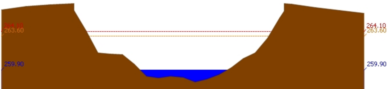
สถานี 070112T แม่น้ำวังที่บ้านบุญนาต ต.บุญนาตพัฒนา อ.เมืองลำปาง จ.ลำปาง ระดับน้ำ 259.90 ม.รทก.
