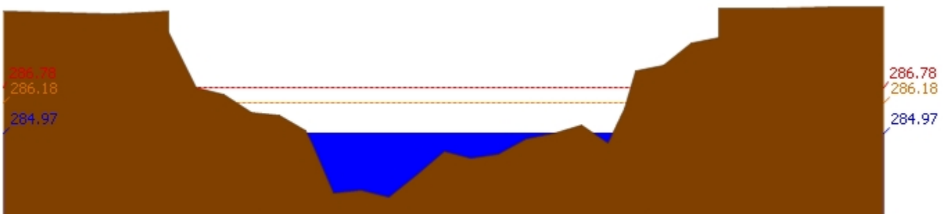
สถานี 070111T แม่น้ำวังที่บ้านแปงโปงชัย ต.บ้านเสา อ.แจ้ห่ม จ.ลำปาง ระดับน้ำ 284.97 ม.รทก.
