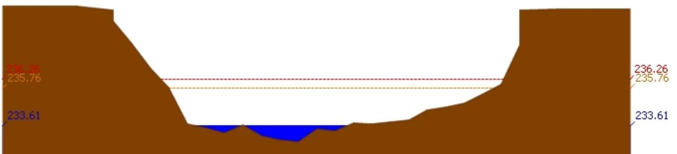
สถานี 070114T แม่น้ำวังที่บ้านปงชัย ต.บ้านเสด็จ อ.เมืองลำปาง จ.ลำปาง ระดับน้ำ 233.61 ม.รทก.
