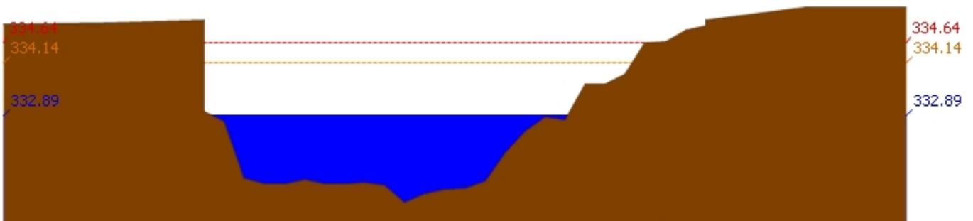
สถานี 070304T น้ำแม่สอยที่บ้านหนองกอก ต.แม่สุก อ.แจ้ห่ม จ.ลำปาง ระดับน้ำ 332.89 ม.รทก.
