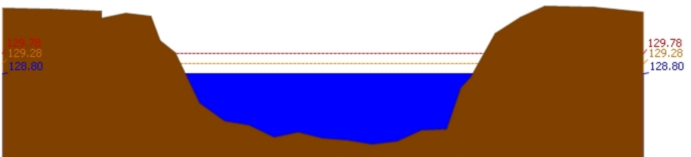
สถานี 070118T แม่น้ำวังที่บ้านแม่สลิด ต.แม่สลิด อ.บ้านตาก จ.ตาก ระดับน้ำ 128.80 ม.รทก.
