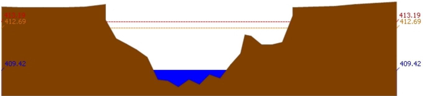
สถานี 070110T แม่น้ำวังที่ อ.วังเหนือ ต.วังเหนือ อ.วังเหนือ จ.ลำปาง ระดับน้ำ 409.42 ม.รทก.
