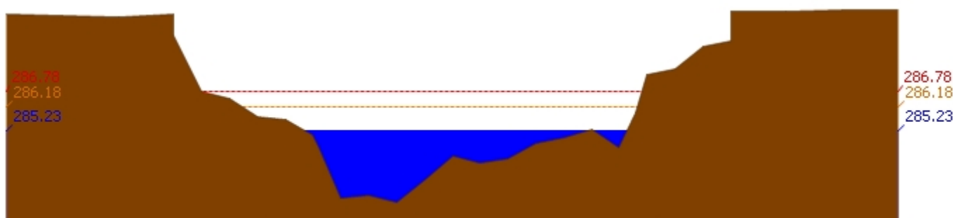
สถานี 070111T แม่บัววังที่บ้านแปงโปงชัย ต.บ้านเสา อ.แจ้ห่ม จ.ลำปาง ระดับน้ำ 285.23 ม.รทก.
