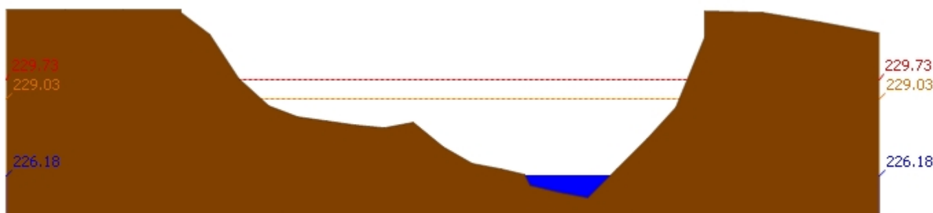
สถานี 070703T น้ำแม่คำที่บ้านนาบอน ต.ทุ่งงาม อ.เสริมงาม จ.ลำปาง ระดับน้ำ 226.18 ม.รทก.
