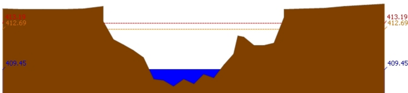
สถานี 070110T แม่น้ำวังที่ อ.วังเหนือ ต.วังเหนือ อ.วังเหนือ จ.ลำปาง ระดับน้ำ 409.45 ม.รทก.
