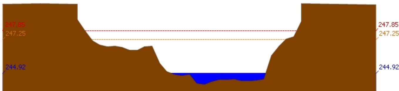
สถานี 070403T น้ำแม่คู่ที่บ้านแค ต.บ้านเป้า อ.เมืองลำปาง จ.ลำปาง ระดับน้ำ 244.92 ม.รทก.
