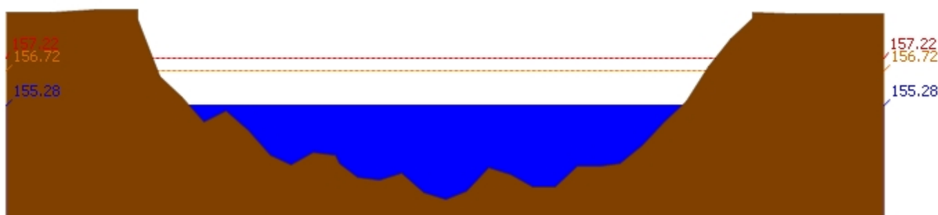
สถานี 070117T แม่น้ำวังที่เทศบาลตำบลแม่ปู ต.แม่ปู อ.แม่พริก จ.ลำปาง ระดับน้ำ 155.28 ม.รทก.
