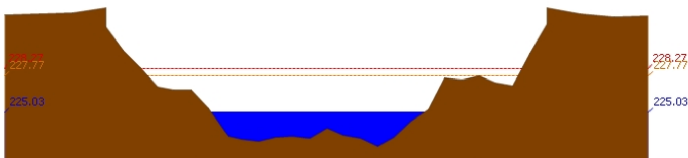
สถานี 070113T แม่น้ำวังที่ จ.ลำปาง ต.เวียงเหนือ อ.เมืองลำปาง จ.ลำปาง ระดับน้ำ 225.03 ม.รทก.
