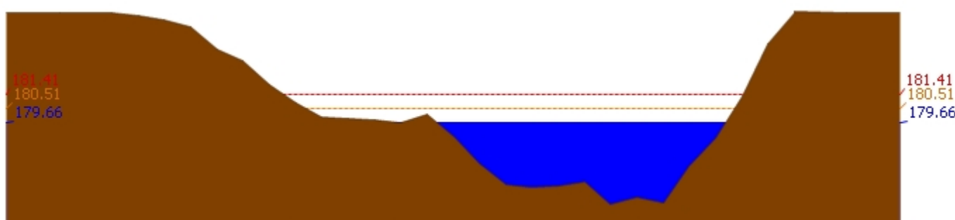
สถานี 070116T แม่น้ำวังที่บ้านแม่เตี๊ยะ ต.แม่ถอด อ.เถิน จ.ลำปาง ระดับน้ำ 179.66 ม.รทก.
