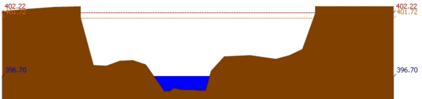
สถานี 060305T น้ำแม่จืดที่บ้านโป่งบัวบาน ต.แม่ปิ้ง อ.พร้าว จ.เชียงใหม่ ระดับน้ำ 396.70 ม.รทก.
