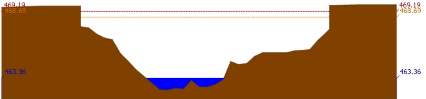
สถานี 060905T น้ำแม่สีที่อำเภอสีคิ้ว อ.สีคิ้ว จ.ลำพูน ระดับน้ำ 463.36 ม.รทก.
