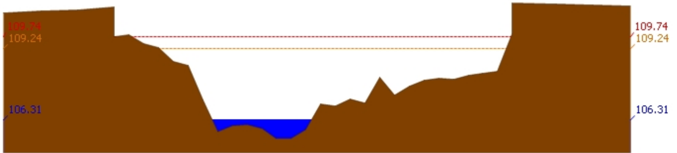
สถานี 061701T ฝายแม่ท้อที่อำเภอเมืองตาก ต.แม่ท้อ อ.เมืองตาก จ.ตาก ระดับน้ำ 106.31 ม.รทก.
