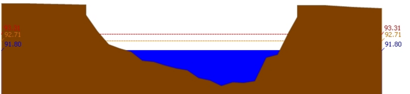
สถานี 061901T คลองแม่ระกาที่บ้านวังชะโอน ต.ท่าไม้ อ.พรานกระต่าย จ.กำแพงเพชร ระดับน้ำ 91.80 ม.รทก.
