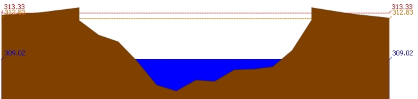
สถานี 060814T น้ำแม่ขานที่บ้านท่าโป่ง ต.บ้านแม อ.สันป่าตอง จ.เชียงใหม่ ระดับน้ำ 309.02 ม.รทก.
