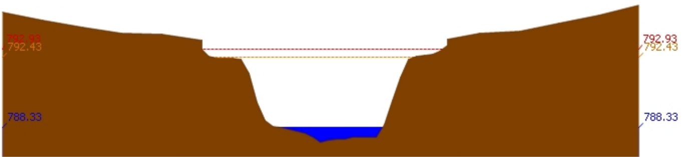
สถานี 061503T น้ำแม่ต้นที่บ้านคอย ต.ยางเปียง อ.อมก๋อย จ.เชียงใหม่ ระดับน้ำ 788.33 ม.รทก.
