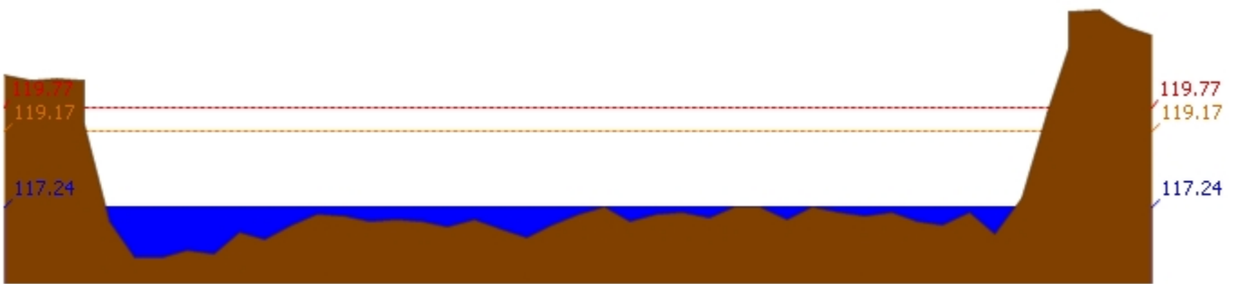
สถานี 060111T แม่น้ำปิงที่บ้านปากร่องห้วยจี่ ต.ตากออก อ.บ้านตาก จ.ตาก ระดับน้ำ 117.24 ม.รทก.
