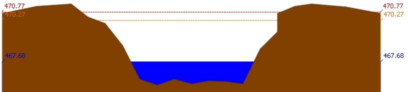
สถานี 061206T น้ำแม่แจ่มที่บ้านทัพ ต.ท่าผา อ.แม่แจ่ม จ.เชียงใหม่ ระดับน้ำ 467.68 ม.รทก.
