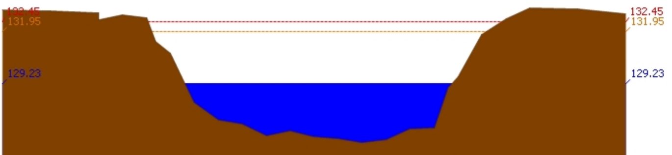
สถานี 070118T แม่น้ำวังที่บ้านแม่สลิด ต.แม่สลิด อ.บ้านตาก จ.ตาก ระดับน้ำ 129.23 ม.รทก.
