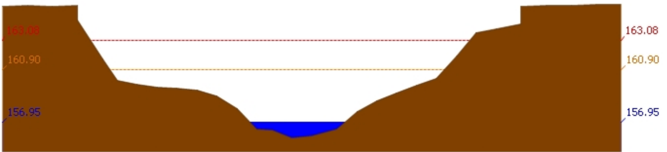
สถานี 120105T แม่น้ำป่าสักที่บ้านวังมเสเหนือ ต.ทำอัญญ อ.หล่มสัก จ.เพชรบูรณ์ ระดับน้ำ 156.95 ม.รทก.
