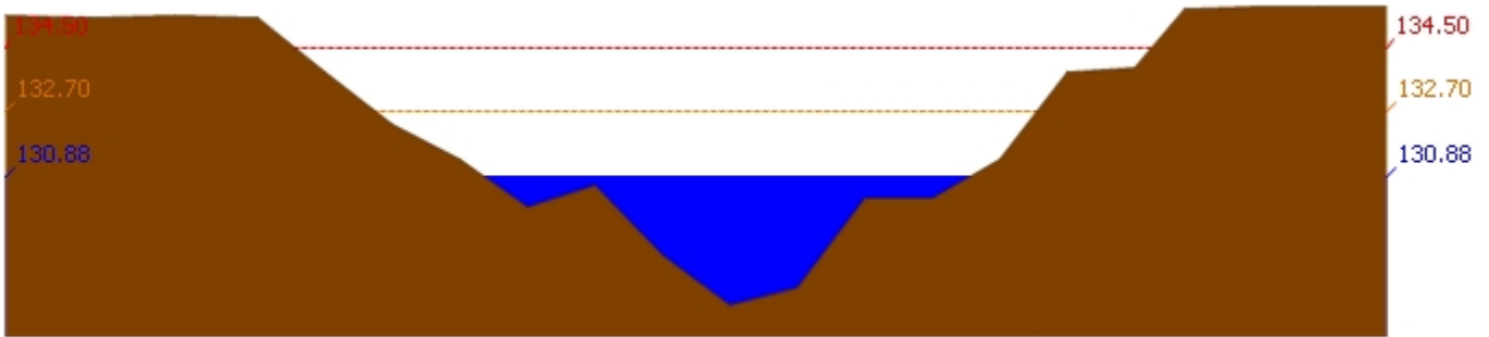
สถานี 120111T แม่น้ำป่าสักที่บ้านจางวาง ต.ลานบัว อ.หล่มสัก จ.เพชรบูรณ์ ระดับน้ำ 130.88 ม.รทก.
