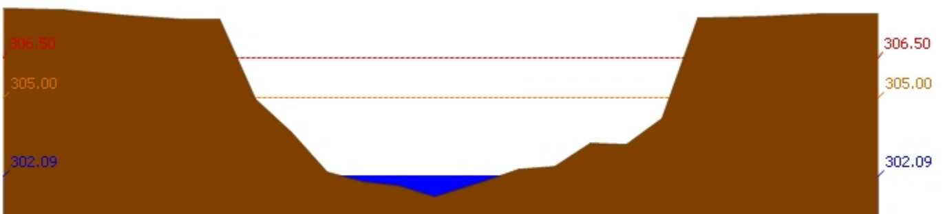
สถานี 120304T หัวน้ำพุที่บ้านกกกะบาก ต.โป่ง อ.ด่านซ้าย จ.เลย ระดับน้ำ 302.09 ม.รทก.
