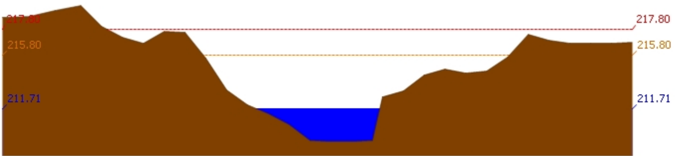
สถานี 120205T แม่น้ำป่าสักที่บ้านอู่กะทาด ต.ศิลา อ.หล่มเก่า จ.เพชรบูรณ์ ระดับน้ำ 211.71 ม.รทก.
