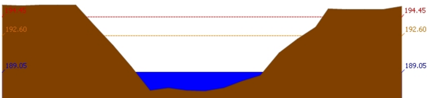
สถานี 120901T ห้วยมวกเหล็กที่ อ.มวกเหล็ก ต.มวกเหล็ก อ.มวกเหล็ก จ.สระบุรี ระดับน้ำ 189.05 ม.รทก.
