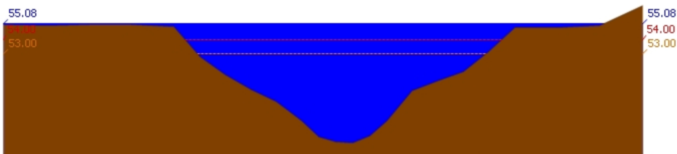
สถานี 120702T ลำสนธิที่บ้านท่าช้าง ต.หนองขาหย่าง อ.ชัยบาดาล จ.ลพบุรี ระดับน้ำ 55.08 ม.รทก.
