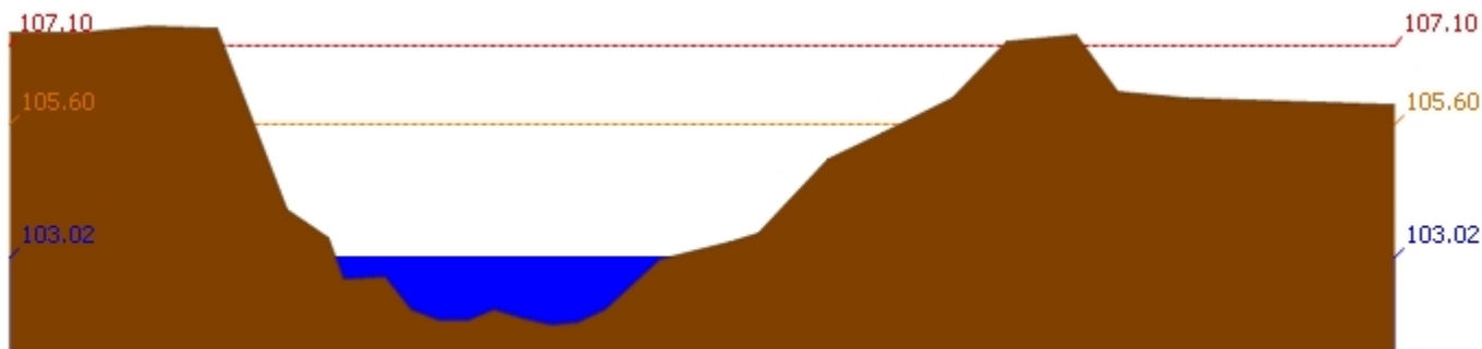
สถานี 110402T ห้วยทับเสลาที่บ้านนาไร่เดียว ต.ลานสัก อ.ลานสัก จ.อุทัยธานี ระดับน้ำ 103.02 ม.รทก.
