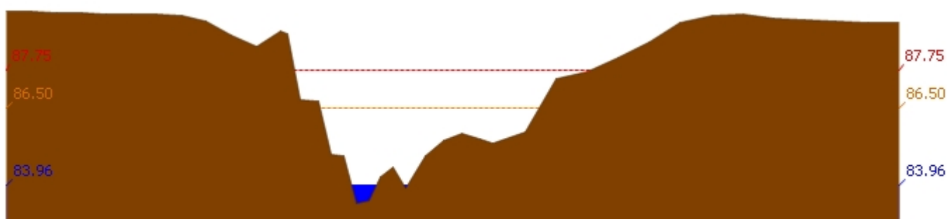
สถานี 110403T ห้วยทับเสลาที่บ้านดินแดง ต.ประดู่ยืน อ.ลานสัก จ.อุทัยธานี ระดับน้ำ 83.96 ม.รทก.
