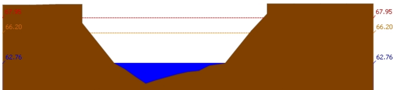
สถานี 110501T น้ำแม่่งที่บ้านคลองสาส์ ต.ลาดยาว อ.ลาดยาว จ.นครสวรรค์ ระดับน้ำ 62.76 ม.รทก.
