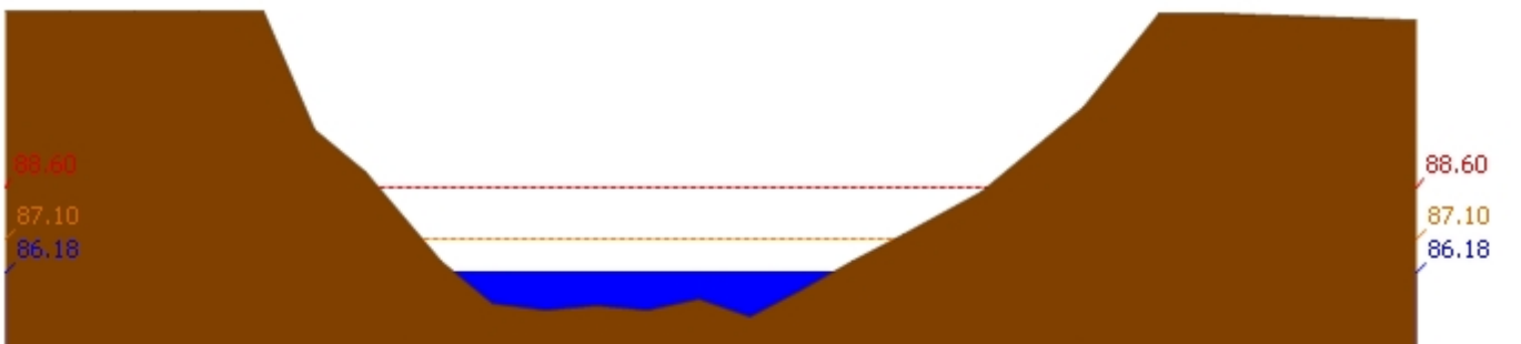
สถานี 120110T แม่น้ำป่าสักที่บ้านวังโบสถ์ ต.วังโบสถ์ อ.หนองไผ่ จ.เพชรบูรณ์ ระดับน้ำ 86.18 ม.รทก.
