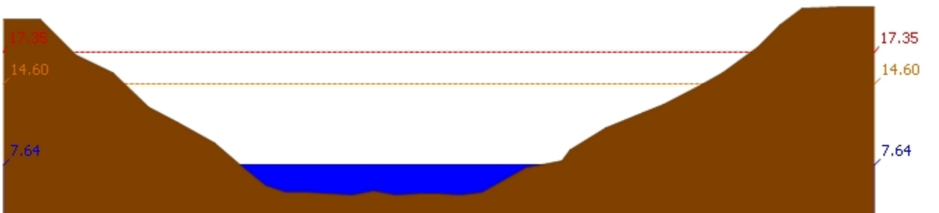
สถานี 120109T แม่น้ำป่าสักที่ อ.แก่งคอย ต.แก่งคอย อ.แก่งคอย จ.สระบุรี ระดับน้ำ 7.64 ม.รทก.
