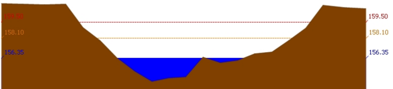
สถานี 120305T หัวเขื่อนป่าสักที่ อ.หล่มเก่า ต.หล่มเก่า อ.หล่มเก่า จ.เพชรบูรณ์ ระดับน้ำ 156.35 ม.รทก.
