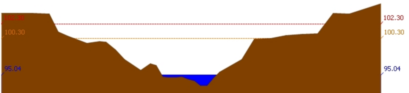
สถานี 120112T แม่น้ำป่าสักที่บ้านหนองแหวน ต.วังมะข่อ อ.เมือง จ.เพชรบูรณ์ ระดับน้ำ 95.04 ม.รทก.
