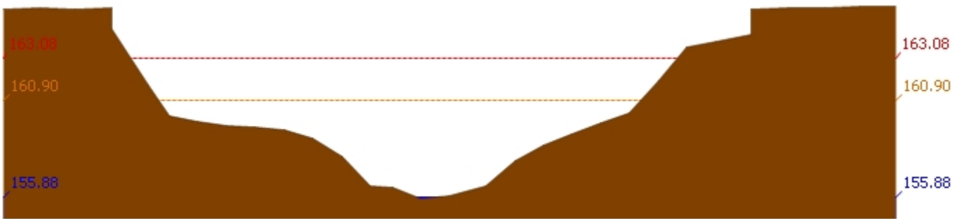
สถานี 120105T แม่น้ำป่าสักที่บ้านวังมเสหนือ ต.ทำอิบุญ อ.หล่มสัก จ.เพชรบูรณ์ ระดับน้ำ 155.88 ม.รทก.
