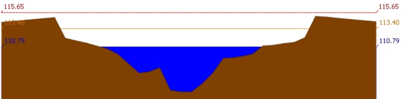
สถานี 120107T แม่น้ำป่าสักที่ อ.เมืองเพชรบูรณ์ ต.นาป่า อ.เมือง จ.เพชรบูรณ์ ระดับน้ำ 110.79 ม.รทก.
