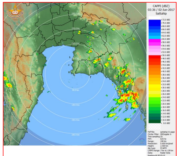
ภาพเรดาร์ตรวจอากาศ “สถานีสัตหีบ” ณ วันที่ 2 มิถุนายน 2560 เวลา 10.36 น. (ที่มา : กรมอุตุนิยมวิทยา)
