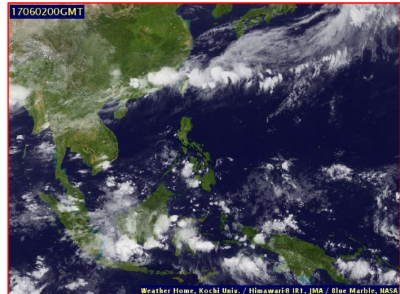
ภาพถ่ายจากดาวเทียม วันที่ 2 มิ.ย. 2560 เวลา 07.00 น.
