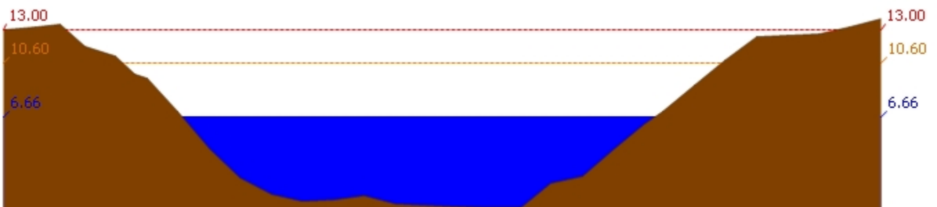
สถานี 120106T แม่น้ำป่าสักที่ อ.เสนาห์ ต.ศาลาวิไทย อ.เสนาห์ จ.สระบุรี ระดับน้ำ 6.66 ม.รทก.
