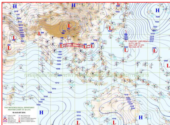
แผนที่อากาศ วันที่ 16 ส.ค. 2559 เวลา 07.00 น.
