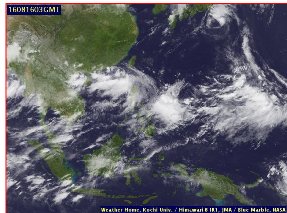
ภาพถ่ายจากดาวเทียม วันที่ 16 ส.ค. 2559
