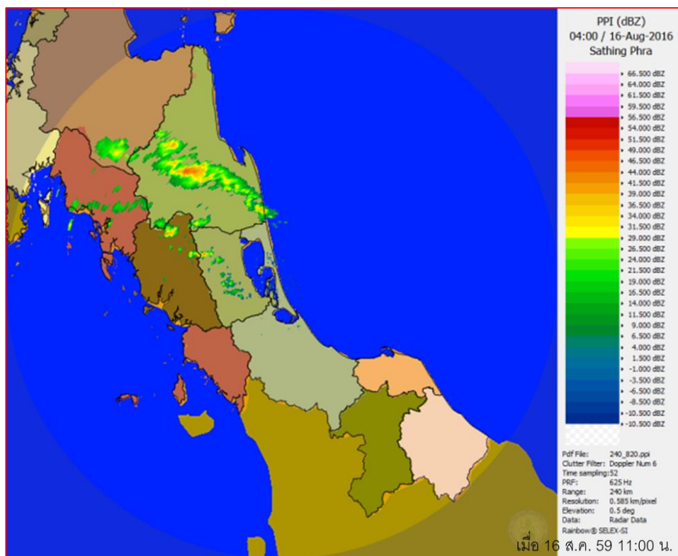
ภาพเรดาร์ตรวจอากาศ “สathingพระ” ณ วันที่ 16 สิงหาคม 2559 (ที่มา : กรมอุตุนิยมวิทยา)
