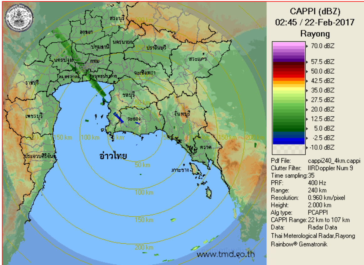
ภาพเรดาร์ตรวจอากาศ “ระยอง” ณ วันที่ 22 กุมภาพันธ์ 2560 (ที่มา : กรมอุตุนิยมวิทยา)
