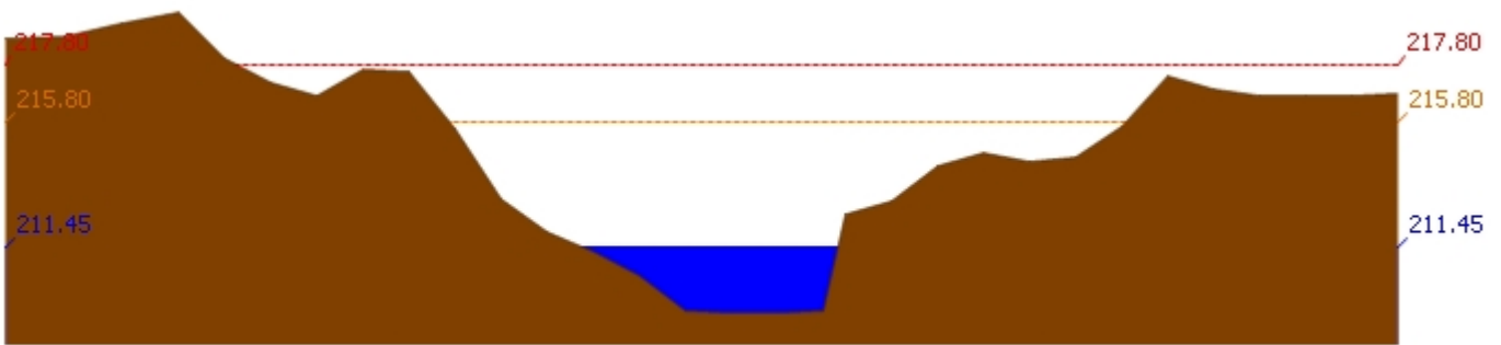
สถานี 120205T แม่น้ำป่าสักที่บ้านอุ้มกะทาด ต.ศิลา อ.หล่มเก่า จ.เพชรบูรณ์ ระดับน้ำ 211.45 ม.รทก.
