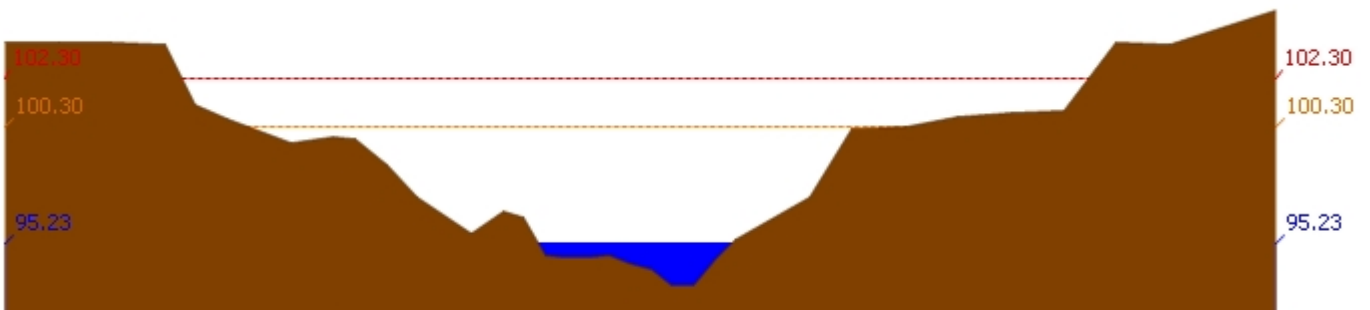
สถานี 120112T แม่น้ำป่าสักที่บ้านหนองแหวน ต.วังมะข่อ อ.เมือง จ.เพชรบูรณ์ ระดับน้ำ 95.23 ม.รทก.
