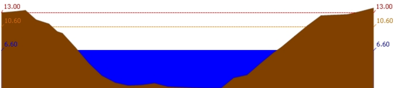
สถานี 120106T แม่น้ำป่าสักที่ อ.เสนาห์ ต.ศาลาวิไทย อ.เสนาห์ จ.สระบุรี ระดับน้ำ 6.60 ม.รทก.
