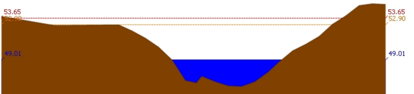
สถานี 120113T แม่น้ำป่าสักที่บ้านเขาค้าง ต.คลองกระจิง อ.ศรีเทพ จ.เพชรบูรณ์ ระดับน้ำ 49.01 ม.รทก.
