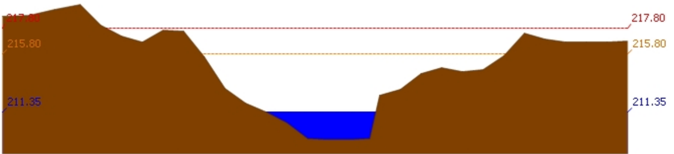
สถานี 120205T แม่น้ำป่าสักที่บ้านอู่กระทัด ต.ศิลา อ.หล่มเก่า จ.เพชรบูรณ์ ระดับน้ำ 211.35 ม.รทก.
