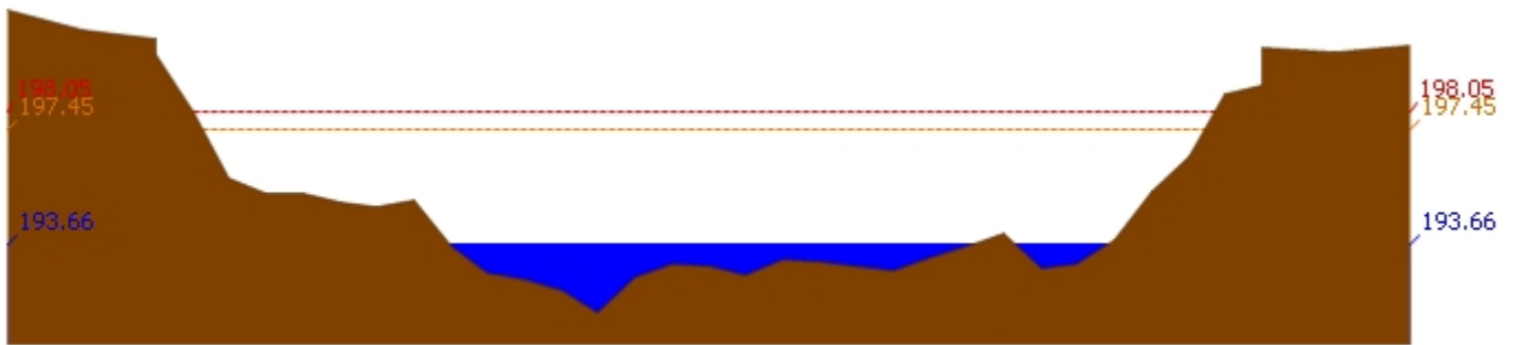
สถานี 070115T น้ำแม่วังที่บ้านอ้อ ต.แม่กัวะ อ.สบปราบ จ.ลำปาง ระดับน้ำ 193.66 ม.รทก.
