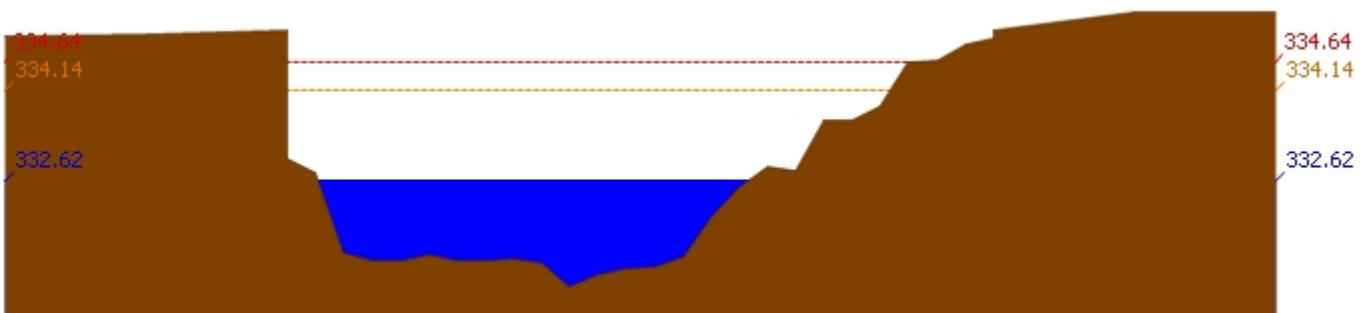
สถานี 070304T น้ำแม่สอยที่บ้านหนองกอก ต.แม่สุก อ.แจ้ห่ม จ.ลำปาง ระดับน้ำ 332.62 ม.รทก.
