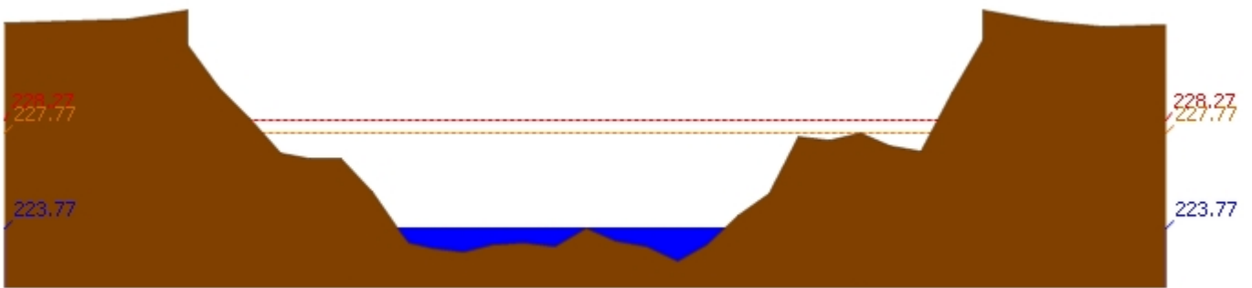
สถานี 070113T แม่น้ำวังที่ จ.ลำปาง ต.เวียงเหนือ อ.เมืองลำปาง จ.ลำปาง ระดับน้ำ 223.77 ม.รทก.
