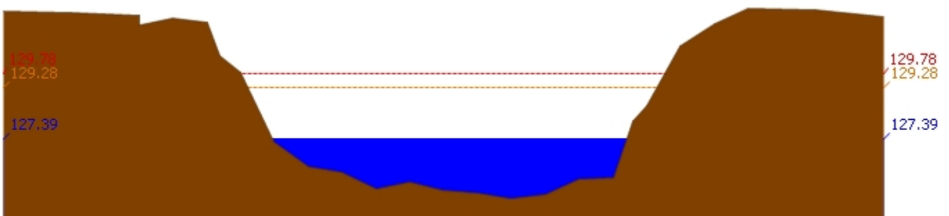
สถานี 070118T แม่น้ำวังที่บ้านแม่สลิด ต.แม่สลิด อ.บ้านตาก จ.ตาก ระดับน้ำ 127.39 ม.รทก.
