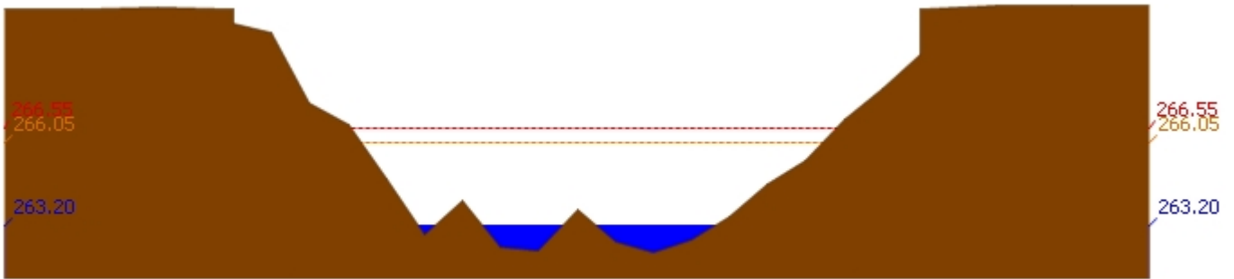
สถานี 070604T น้ำแม่จางที่บ้านสุโหมไชยมงคล ต.หัวเสือ อ.แม่ทะ จ.ลำปาง ระดับน้ำ 263.20 ม.รทก.
