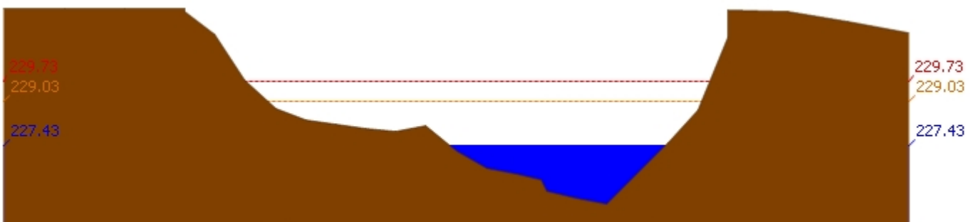
สถานี 070703T น้ำแม่ตำที่บ้านนาบอน ต.ทุ่งงาม อ.เสริมงาม จ.ลำปาง ระดับน้ำ 227.43 ม.รทก.
