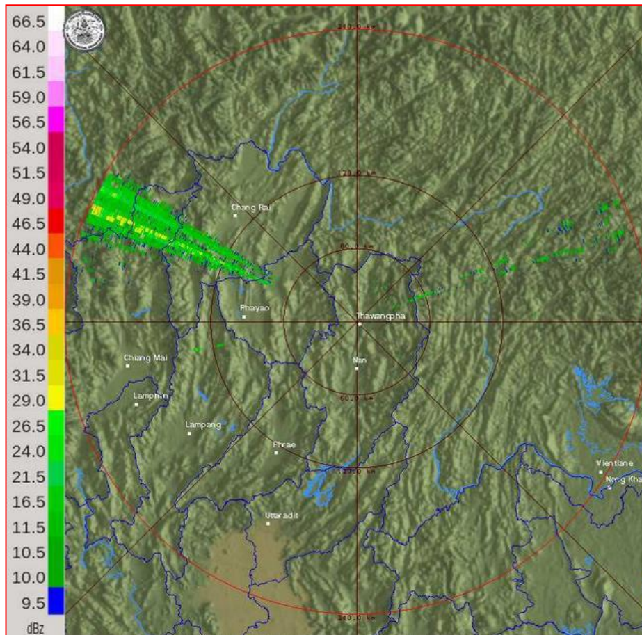
ภาพเรดาร์ตรวจอากาศ “น่าน” ณ วันที่ 16 มีนาคม 2560 (ที่มา : กรมอุตุนิยมวิทยา)
