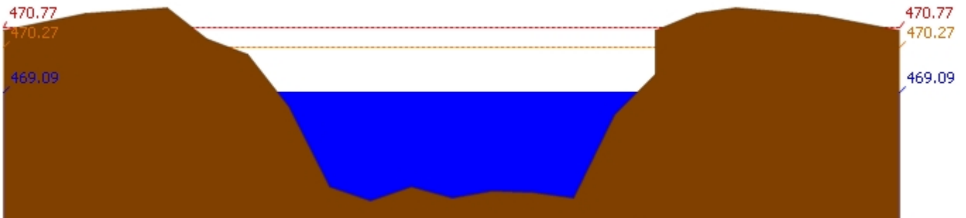
สถานี 061206T น้ำแม่แจ่มที่บ้านทัพ ต.ท่าผา อ.แม่แจ่ม จ.เชียงใหม่ ระดับน้ำ 469.09 ม.รทก.
