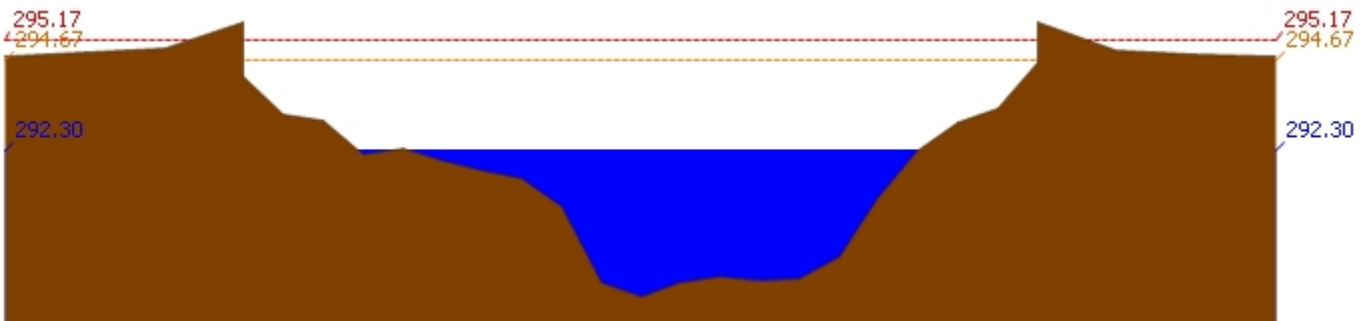
สถานี 060709T น้ำแม่กวังที่ลำพูน ต.เวียงของ อ.เมือง จ.ลำพูน ระดับน้ำ 292.30 ม.รทก.
