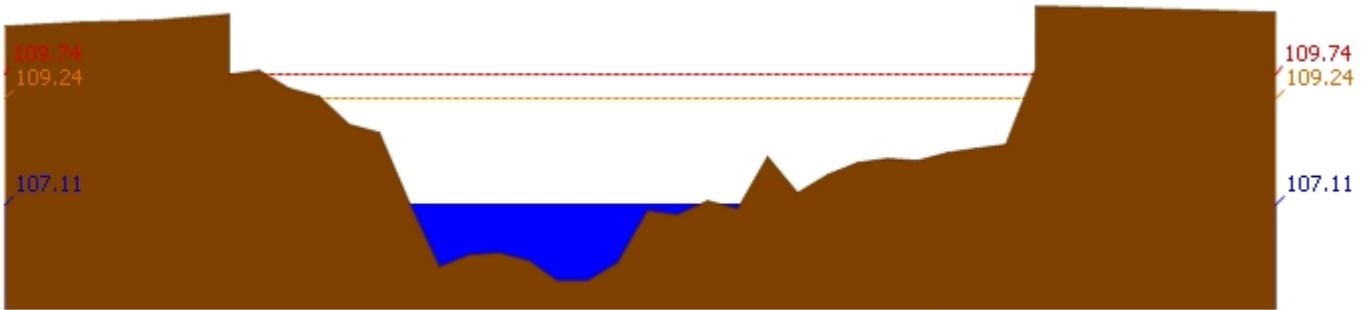
สถานี 061701T ฝายแม่ท้อที่อำเภอเมืองตาก ต.แม่ท้อ อ.เมืองตาก จ.ตาก ระดับน้ำ 107.11 ม.รทก.
