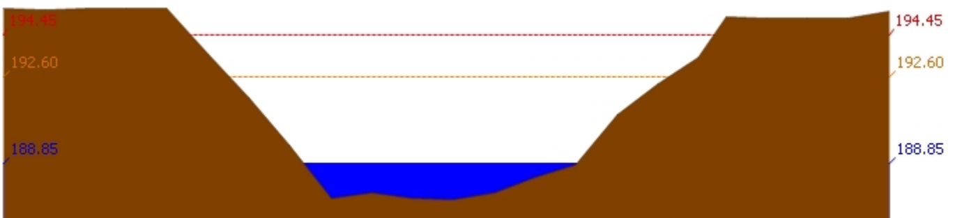
สถานี 120901T ห้วยมวกเหล็กที่ อ.มวกเหล็ก ต.มวกเหล็ก อ.มวกเหล็ก จ.สระบุรี ระดับน้ำ 188.85 ม.รทก.
