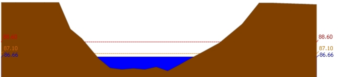
สถานี 120110T แม่น้ำป่าสักที่บ้านวังโบสถ์ ต.วังโบสถ์ อ.หนองไผ่ จ.เพชรบูรณ์ ระดับน้ำ 86.66 ม.รทก.
