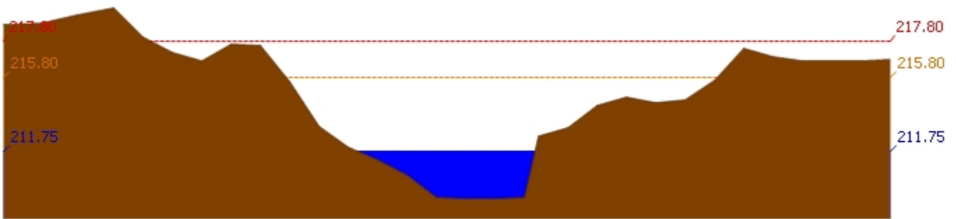
สถานี 120205T แม่น้ำป่าสักที่บ้านอู่กะทาด ต.ศิลา อ.หล่มเก่า จ.เพชรบูรณ์ ระดับน้ำ 211.75 ม.รทก.
