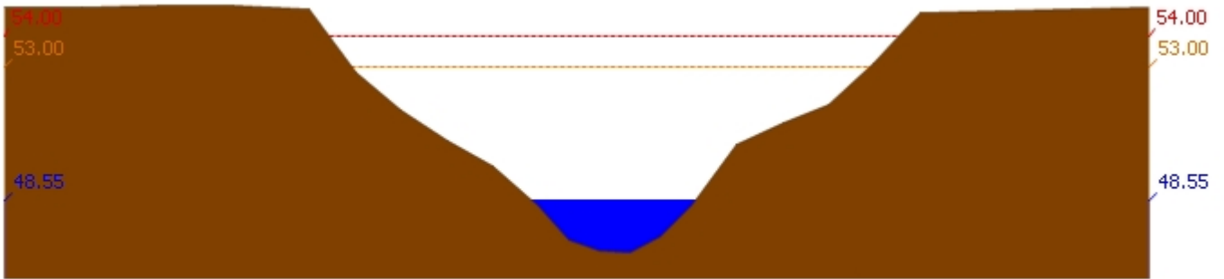
สถานี 120702T ลำสนธิที่บ้านท่าช้าง ต.หนองขาหย่าง อ.ชัยบาดาล จ.ลพบุรี ระดับน้ำ 48.55 ม.รทก.
