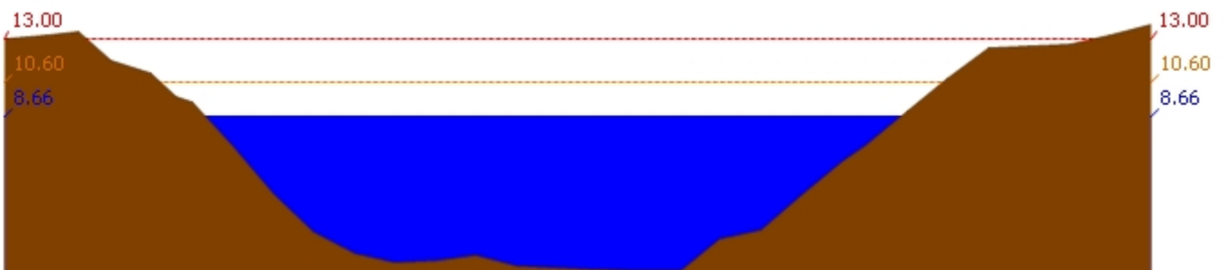
สถานี 120106T แม่น้ำป่าสักที่ อ.เสนาห์ ต.ศาลาวิไทย อ.เสนาห์ จ.สระบุรี ระดับน้ำ 8.66 ม.รทก.
