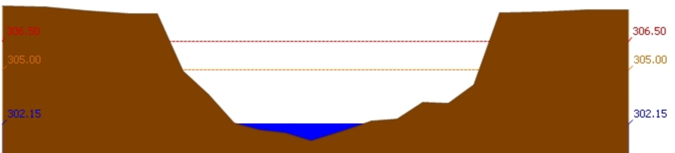
สถานี 120304T หัวน้ำพุที่บ้านกกกะบาก ต.โป่ง อ.ด่านซ้าย จ.เลย ระดับน้ำ 302.15 ม.รทก.
