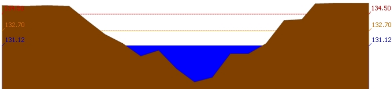
สถานี 120111T แม่น้ำป่าสักที่บ้านจางวาง ต.ลานบัว อ.หล่มสัก จ.เพชรบูรณ์ ระดับน้ำ 131.12 ม.รทก.
