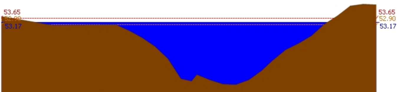
สถานี 120113T แม่น้ำป่าสักที่บ้านเขาค้าง ต.คลองกระจิง อ.ศรีเทพ จ.เพชรบูรณ์ ระดับน้ำ 53.17 ม.รทก.
