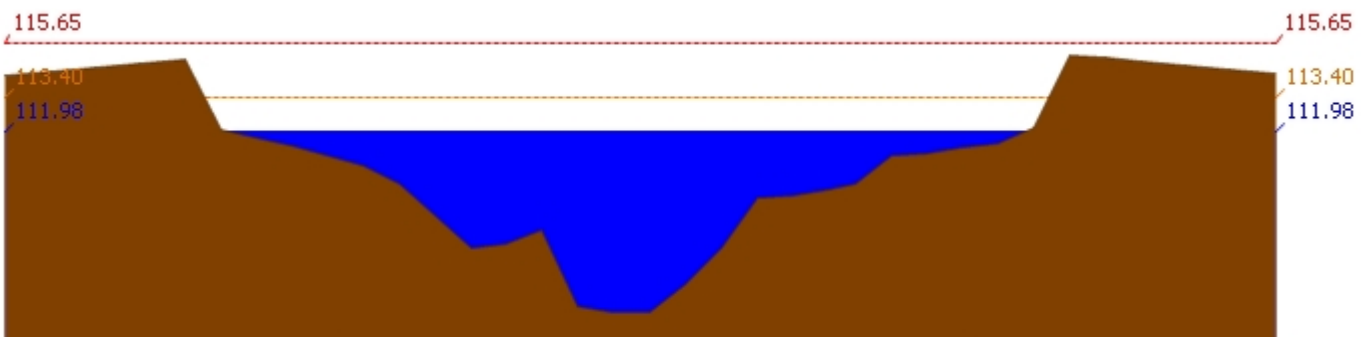
สถานี 120107T แม่น้ำป่าสักที่ อ.เมืองเพชรบูรณ์ ต.นาป่า อ.เมือง จ.เพชรบูรณ์ ระดับน้ำ 111.98 ม.รทก.
