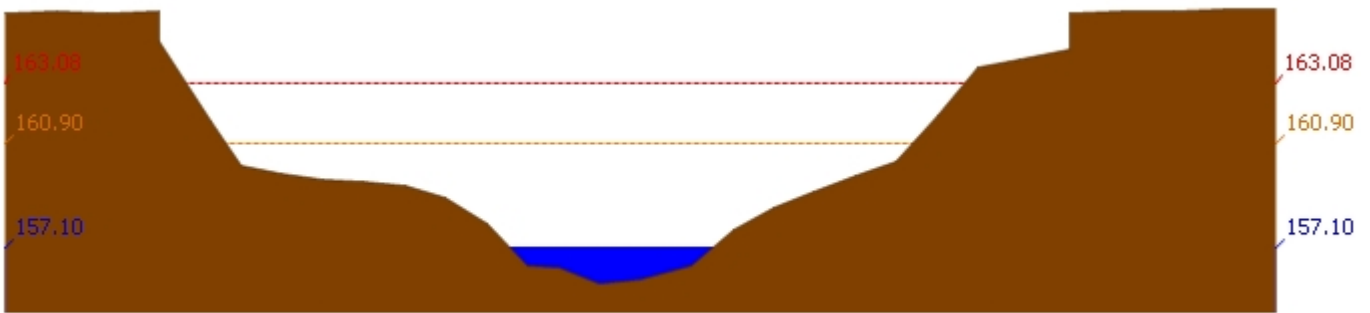
สถานี 120105T แม่น้ำป่าสักที่บ้านวังมเหนื่อ ต.ทำอัญญา อ.หล่มสัก จ.เพชรบูรณ์ ระดับน้ำ 157.10 ม.รทก.
